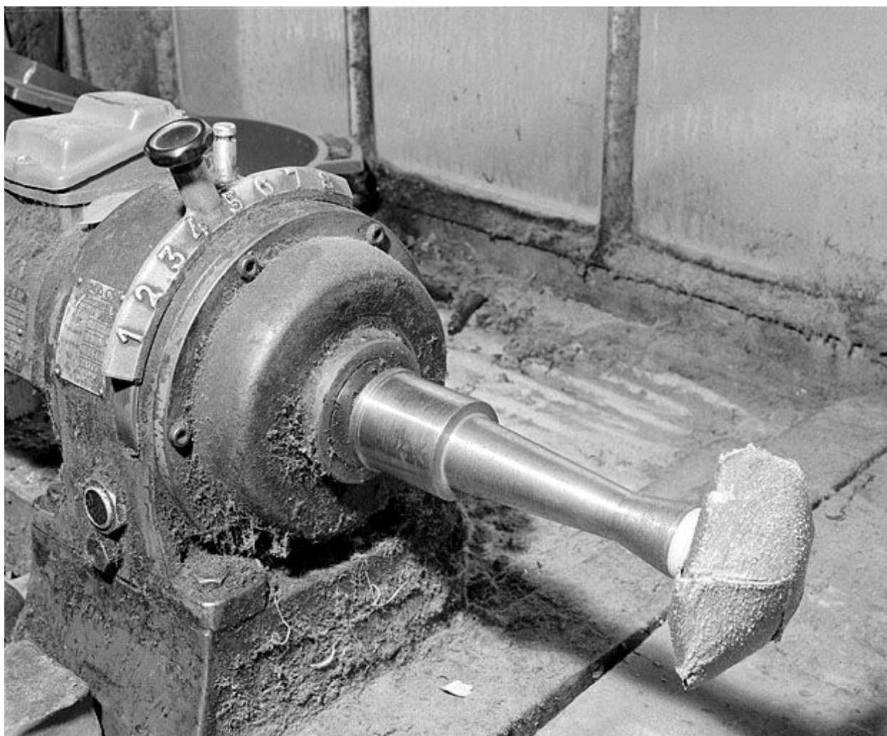
Vue rapprochée : variateur et disque de polissage.
