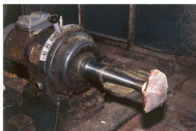
Vue rapprochée : variateur et disque de polissage. Phot. Jérôme Mongreville IVR43_20003900987ZA
