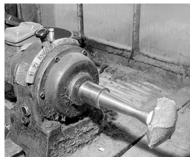
Vue rapprochée : variateur et disque de polissage. Phot. Jérôme Mongreville IVR43_20003900986X
