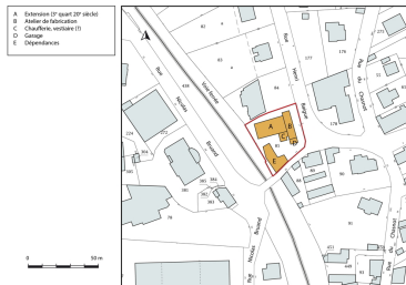
Plan-masse et de situation. Extrait du plan cadastral, 2019. Dess. Bertrand Turina IVR43_20192501099NUDA
