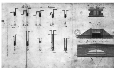
Usine de Mr Tinseau. Instruction des réclamations formulées par la commune de Valay contre la retenue du haut fourneau de Valay, [profil en travers et ouvrages d'art]. Phot. Jérôme Mongreville IVR43_19877000082X
