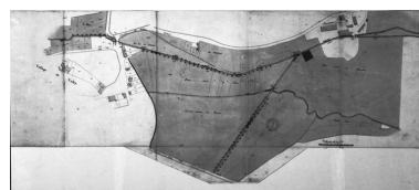
Usine de Mr Tinseau. Instruction des réclamations formulées par la commune de Valay contre la retenue du haut fourneau de Valay, [plan-masse et de situation]. Phot. Jérôme Mongreville IVR43_19877000083X
