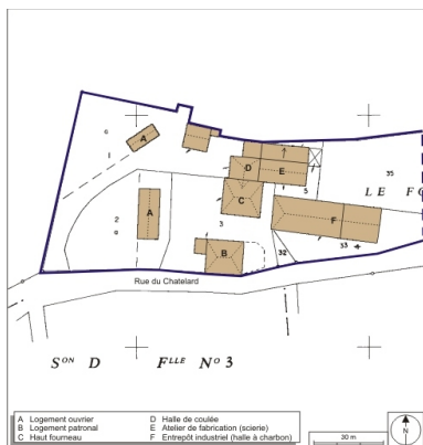
Plan-masse et de situation. Extrait du plan cadastral numérisé, 2008, section AD, 1:1000. Source : Direction
