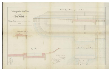
Barrage avec pertuis à construire en amont de la dérivation d'Auxonne. [Plan, coupe et élévation]. 1840. Phot. Petot Frédéric, Phot. Thierry Kuntz IVR26_20202100091NUC4AQ
