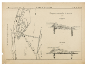
Barrage d'Auxonne. Plan général du barrage et de ses abords. Coupes. 1886.
