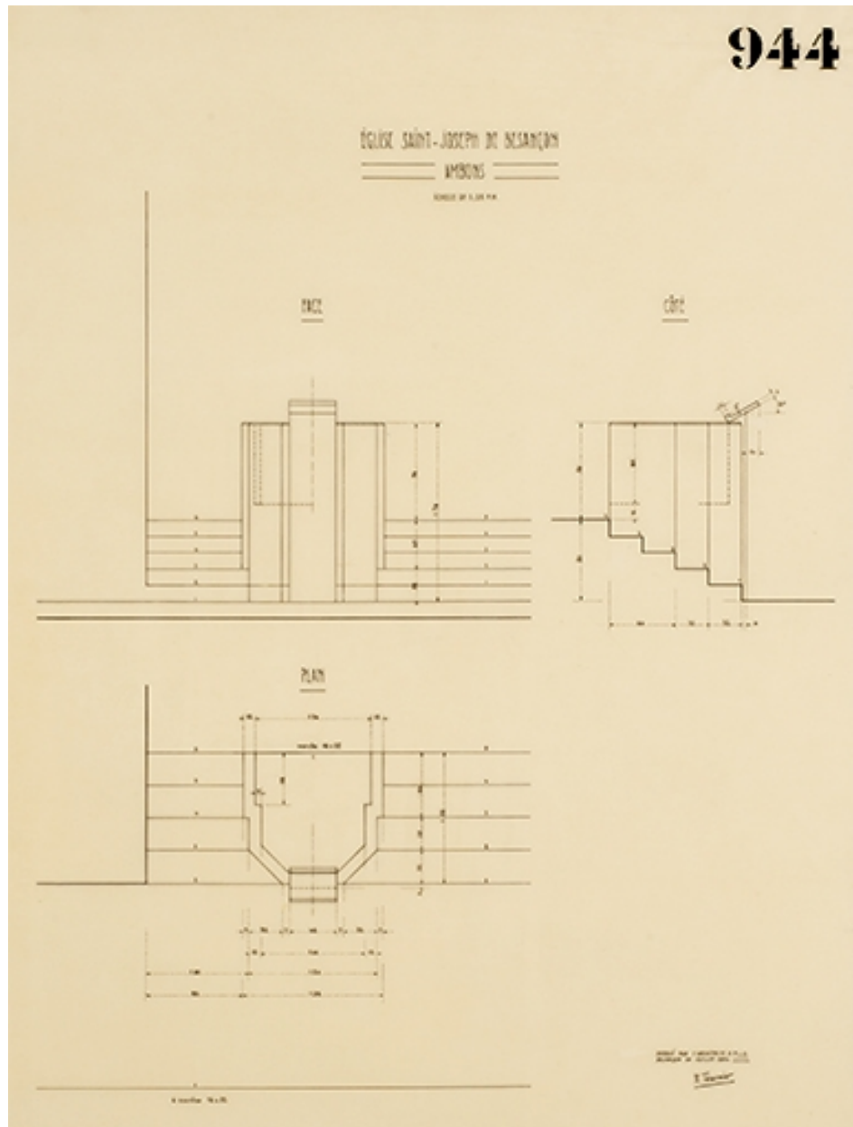
Plan et élévations des ambons de l'église Saint-Joseph. Juillet 1954.
