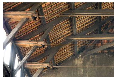
Atelier de fonderie. Détail des étriers de la charpente. Phot. Jérôme Mongreville IVR43_20087000725NUC2A
