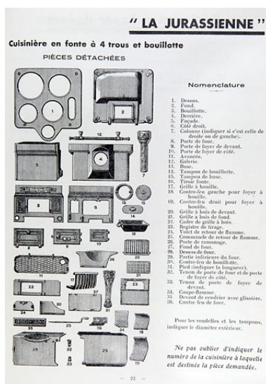
Pièces détachées de la cuisinière La Jurassienne. Phot. Jérôme Mongreville IVR43_20097000014NUC2A
