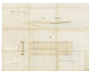
Dessin d'un bac à construire pour le passage de la Saône au Port-Saint-Pierre. [Plan, coupes et élévation]. 1849
