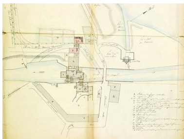
Plan des forges, fourneau, moulin de Seveux à Mr le duc De Marmier [détail]. Phot. Jérôme Mongreville, Autr. Guyet IVR43_20097000024NUC2A
