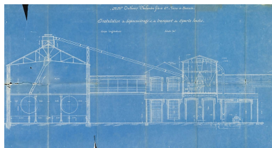
MM. Outhenin-Chalandre Fils et Cie. Usine de Seveux. Installation de dépoussiérage et de transport du sparte haché, coupe longitudinale. Phot. Jérôme Mongreville IVR43_20097000048NUC2A
