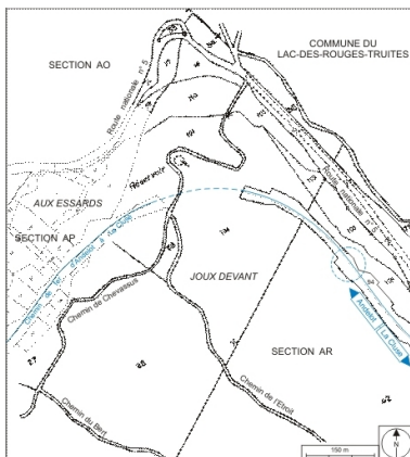
Plan-masse et de situation. Montage d'extraits du plan cadastral informatisé, 2006, sections AP et AR, échelle 1:5000. Dess. André Céréza IVR43_20073900229NUDA
