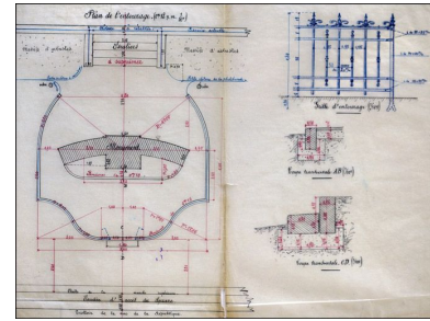
Entourage du Monument commémoratif. Bordures et Grilles : dessin sur calque (plume), 6 novembre 1922, échelles 1:50 (plan) et 1:10 (coupes et élévation). Phot. Yves Sancey, Autr. NEPASUTILISERLacroix (architecte voyer) IVR43_20103900049NUC2A
