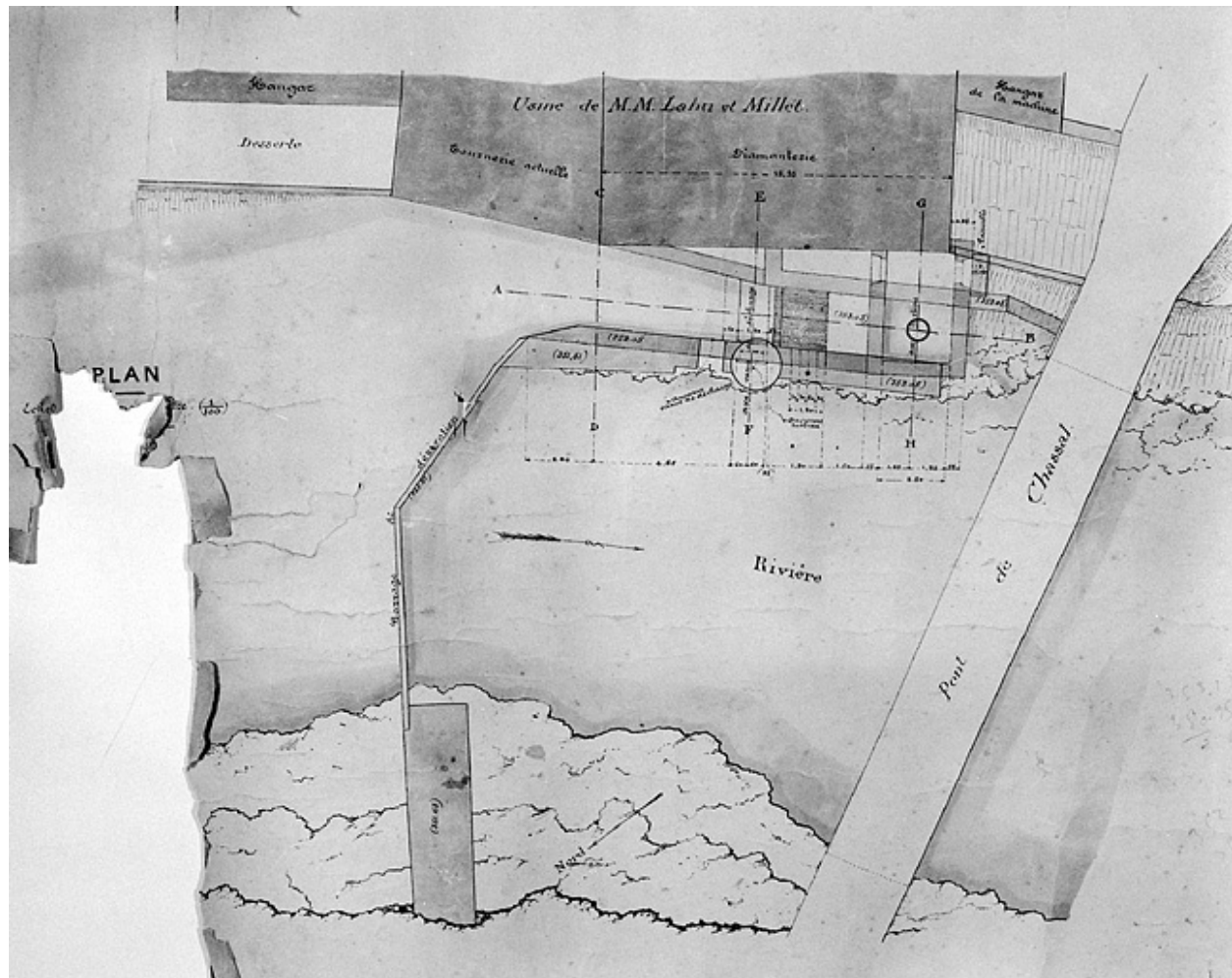
Plan, coupes et élévation de l'usine de MM Millet et Lahu [...], détail du plan.
