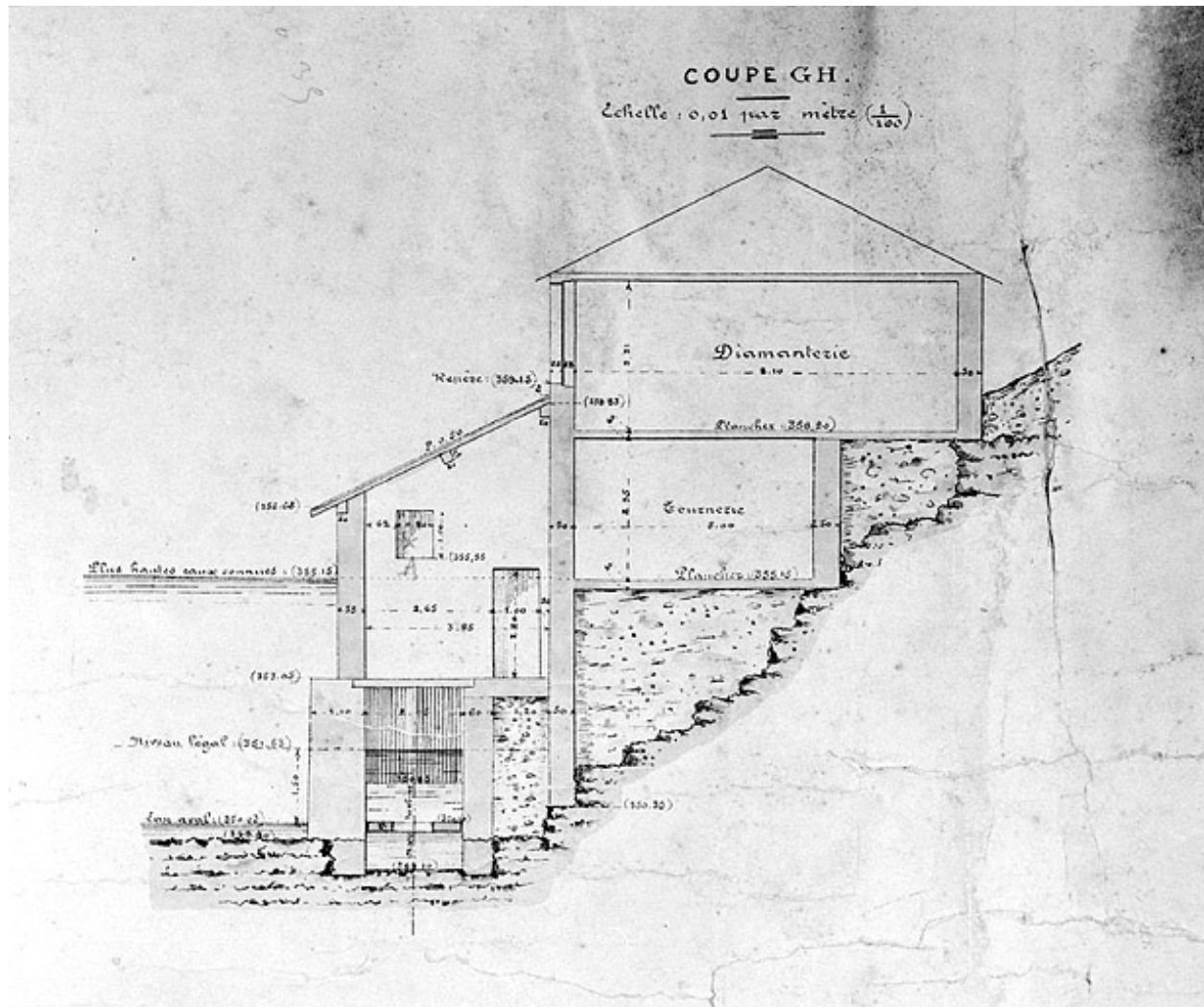
Plan, coupes et élévation de l'usine de MM Millet et Lahu [...], coupe transversale.
