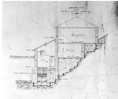
Plan, coupes et élévation de l'usine de MM Millet et Lahu [...], coupe transversale. Phot. Jérôme Mongreville IVR43_19903900359X
