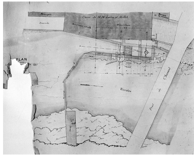
Plan, coupes et élévation de l'usine de MM Millet et Lahu [...], détail du plan. Phot. Jérôme Mongreville IVR43_19903900358X
