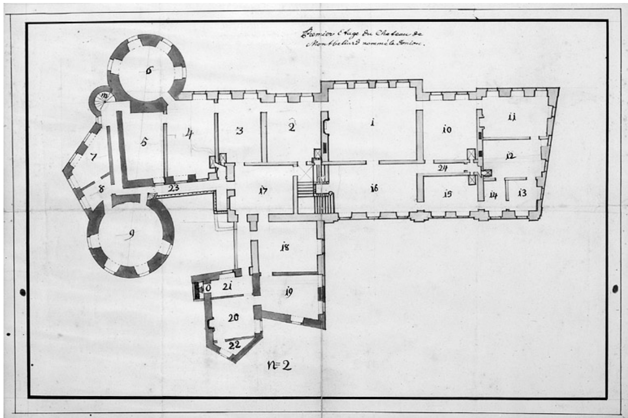
Projet de reconstruction de l'aile principale. Plan du premier étage, 1750.
