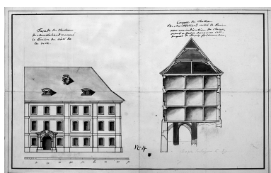
Projet de reconstruction de l'aile principale. Elévation de la façade sur cour et coupe du bâtiment, 1750. Phot. Jérôme Mongreville, Autr. Anthonus (?) Schrotz IVR43_19872500249V
