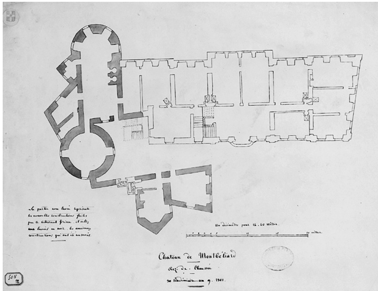
Château de Montbéliard. Plan du rez-de-chaussée, 1801.
