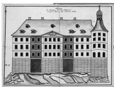
Projet de reconstruction de l'aile principale. Elévation de la façade sud, 1750. Phot. Jérôme Mongreville, Autr. Anthonus (?) Schrotz IVR43_19872500405V
