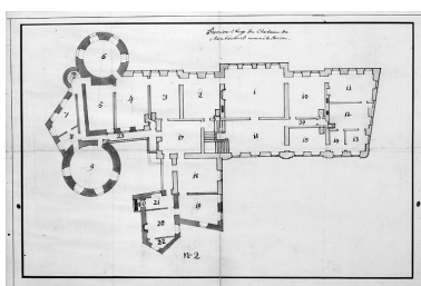
Projet de reconstruction de l'aile principale. Plan du premier étage, 1750. Phot. Jérôme Mongreville, Autr. Anthonus (?) Schrotz IVR43_19872500247V
