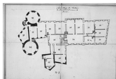
Projet de reconstruction de l'aile principale. Plan du second étage, 1750. Phot. Jérôme Mongreville, Autr. Anthonus (?) Schrotz IVR43_19872500248X
