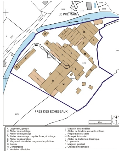
Plan-masse et de situation. Extrait du plan cadastral numérisé, 2008, section A, 1:1250. Source : Direction générale des Finances Publiques - Cadastre ; mise à jour : 2008. Dess. André Céréza IVR43_20087000389NUDA
