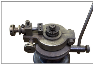
Partie supérieure de la machine à ménisquer Cathenoz. Phot. Yves Sancey IVR43_20103900275NUC2A
