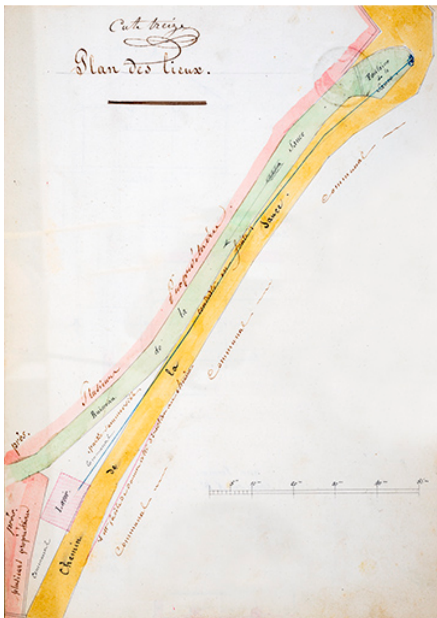
Plan des lieux [pour la construction de la fontaine-lavoir de la Sauce à Scey-sur-Saône-et-Saint-Albin]. 1848.
