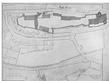
Plan parcellaire de 1859, feuille 9. Phot. Jérôme Mongreville, Autr. Ad. Pawlowski IVR43_19862500516V
