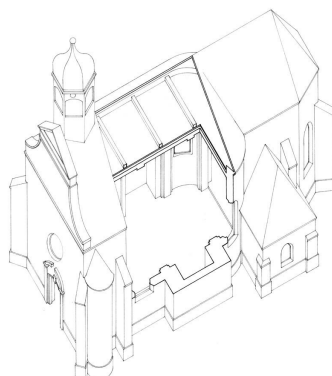
coupe axonométrique Dess. Alain Morelière IVR26_20122100803A2YY
