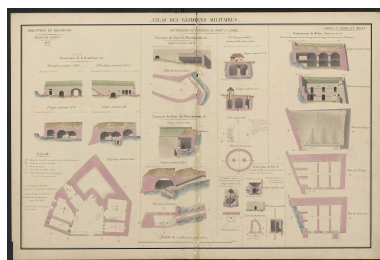
Atlas des bâtiments militaires. Direction de Besançon. Place de Salins. Forts St-André et Belin. 1835. La demi-lune est représentée sur les colonnes de gauche et du centre. Autr. auteur inconnu IVR43_20223901188NUC4A
