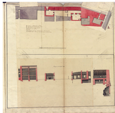
Fol. 16 Fort-Belin-sur-Salins : plans et coupes (magasin pour 12,000 milliers de poudre) - vue 2. IVR43_20243900507NUC4A
