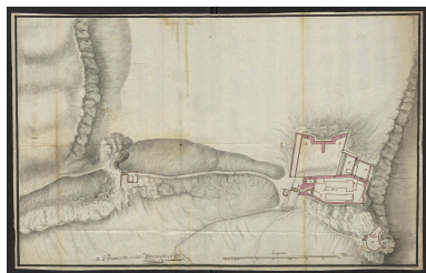
Plan du fort Belin de Salins. 30 novembre 1698. Autr. Isaac Robelin IVR43_20213900169NUC4A
