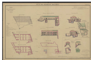
Place de Salins. Fort Belin. Réduit - côté A au plan général. 1848. IVR43_20223901189NUC4A
