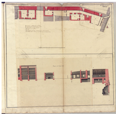
Fol. 16 Fort-Belin-sur-Salins : plans et coupes (magasin pour 12,000 milliers de poudre) - vue 1. IVR43_20243900506NUC4A
