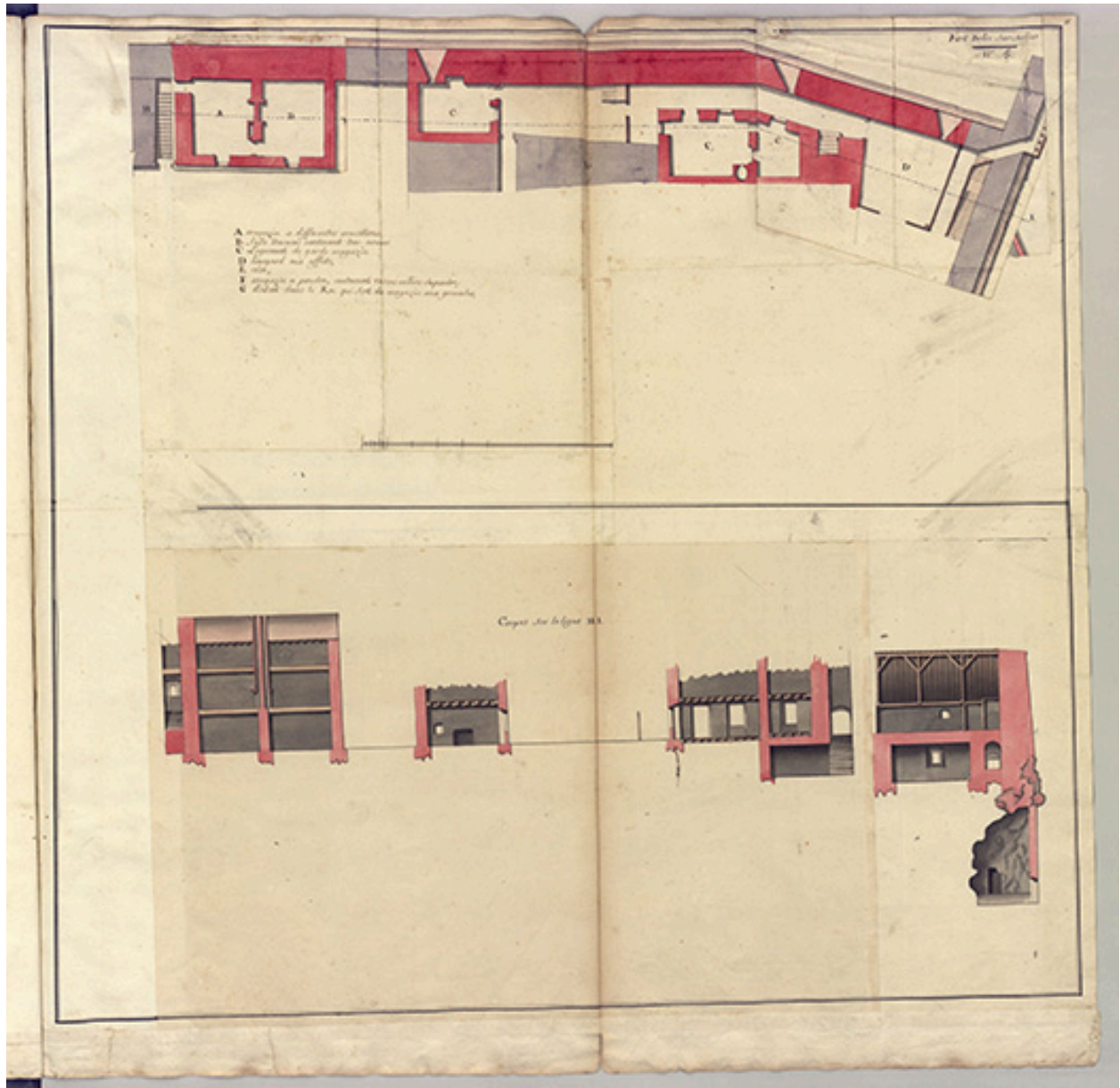
Fol. 16 Fort-Belin-sur-Salins : plans et coupes (magasin pour 12,000 milliers de poudre) - vue 1.
