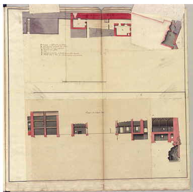
Fol. 16 Fort-Belin-sur-Salins : plans et coupes (magasin pour 12,000 milliers de poudre) - vue 3. IVR43_20243900508NUC4A
