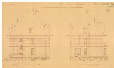
Monsieur Carrel F., rue Delavelle à Besançon. Projet de construction d'une villa. Façade latérale ouest [et] Façade postérieure, 1928. Autr. Pierre Noë IVR43_20152500124NUC2A
