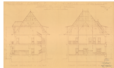
Monsieur Carrel F., rue Delavelle à Besançon. Projet de construction d'une villa. Coupe parallèle à la rue [et] Coupe perpendiculaire à la rue, 1928. Autr. Pierre Noë IVR43_20152500122NUC2A
