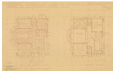
Monsieur Carrel F., rue Delavelle à Besançon. Projet de construction d'une villa. Plan du rez-de-chaussée [et] Plan du premier étage, 16 octobre 1928. Autr. Pierre Noë IVR43_20152500121NUC2A
