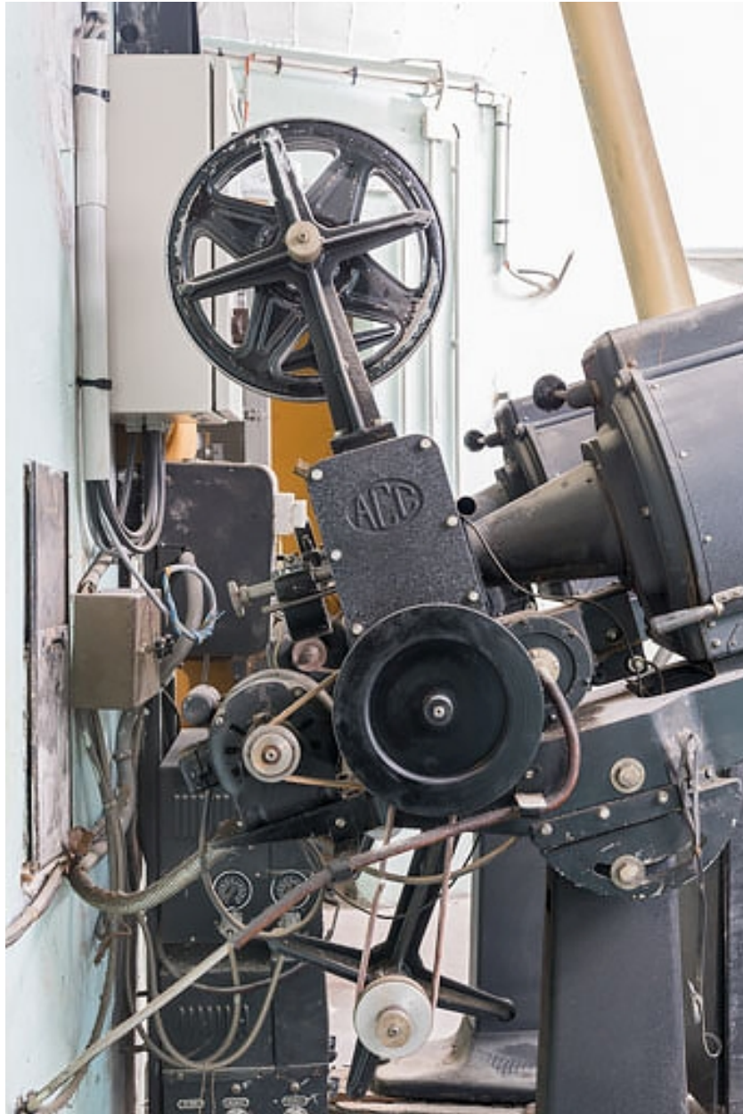
Projecteur côté jardin : système d'entraînement du film et supports des bobines.
