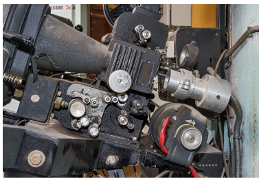
Projecteur côté cour : système d'entraînement du film et objectif. Phot. Pierre-Marie Barbe-Richaud IVR26_20222100050NUC4A
