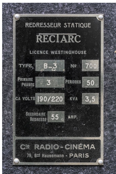
Redresseur Rectarc désaffecté : plaque de constructeur. Phot. Pierre-Marie Barbe-Richaud IVR26_20222100063NUC4A
