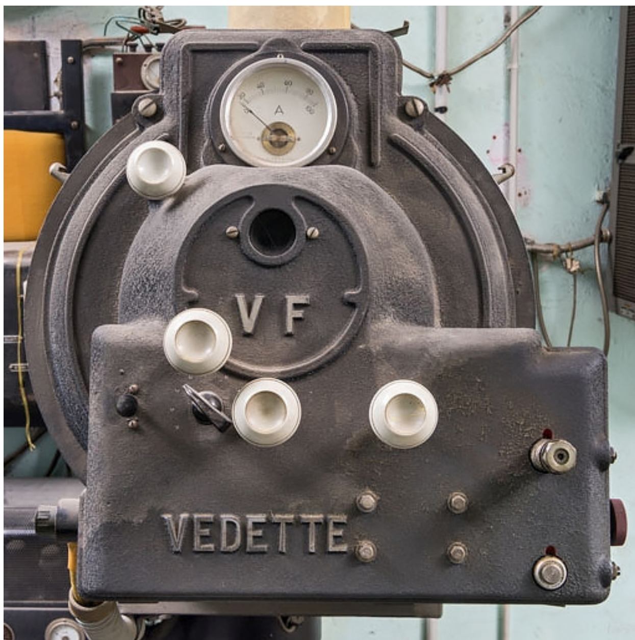
Projecteur côté cour : arrière de la lanterne.
