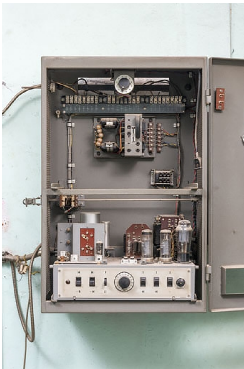
Armoire de commande Philips, porte ouverte.
