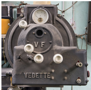
Projecteur côté cour : arrière de la lanterne. Phot. Pierre-Marie Barbe-Richaud IVR26_20222100051NUC2A
