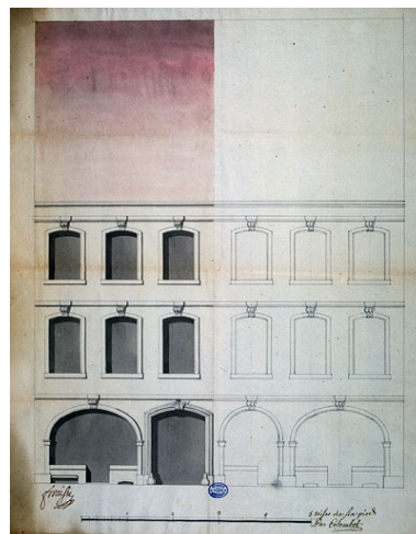
Élévation de la partie gauche de la façade sur rue. Dessin à la plume aquarellé, s.d. (1755).
