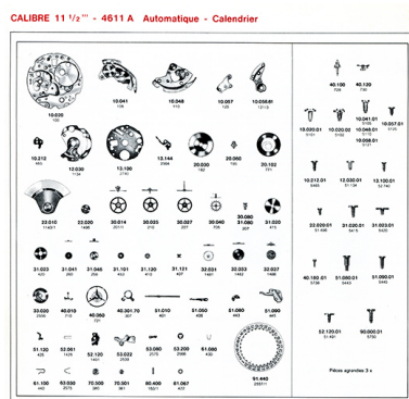
Calibre 11 1/2''' - 4611 A Automatique Calendrier [éclaté des fournitures], 1973. Autr. auteur inconnu IVR43_20162500140NUC2A
