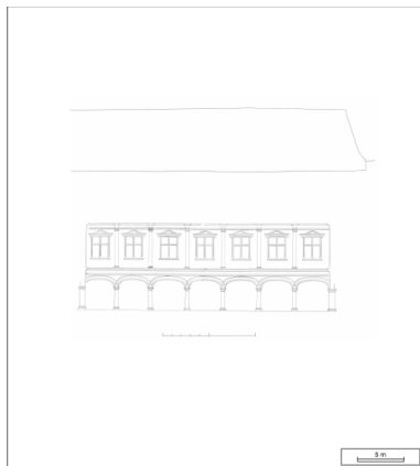
Restitution photogrammétrique de l'élévation externe de la façade sud sur cour intérieure. Dessin original numérique, 2002 Dess. André Céréza, Autr. Michel Andry IVR43_20092501243NUD
