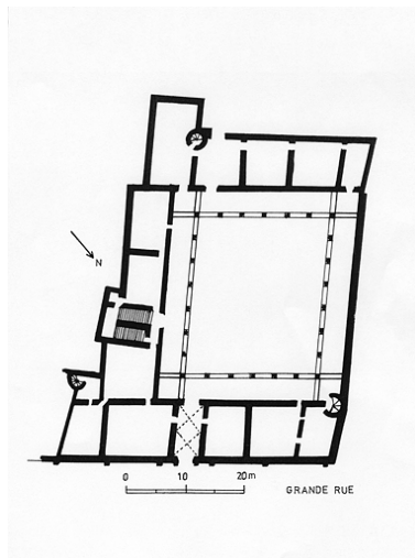
Plan du rez-de-chaussée d'après le relevé de Bérard en 1872. Dessin, fin du 20e siècle. Phot. Yves Sancey IVR43_20092501247NUC2A
