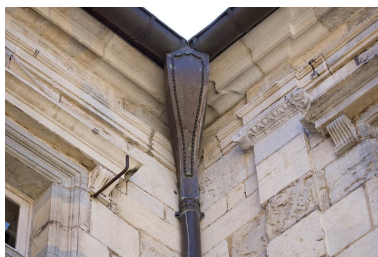
Détail d'une cuvette pour la descente des eaux. Phot. Yves Sancey IVR43_20092501030NUC2A
