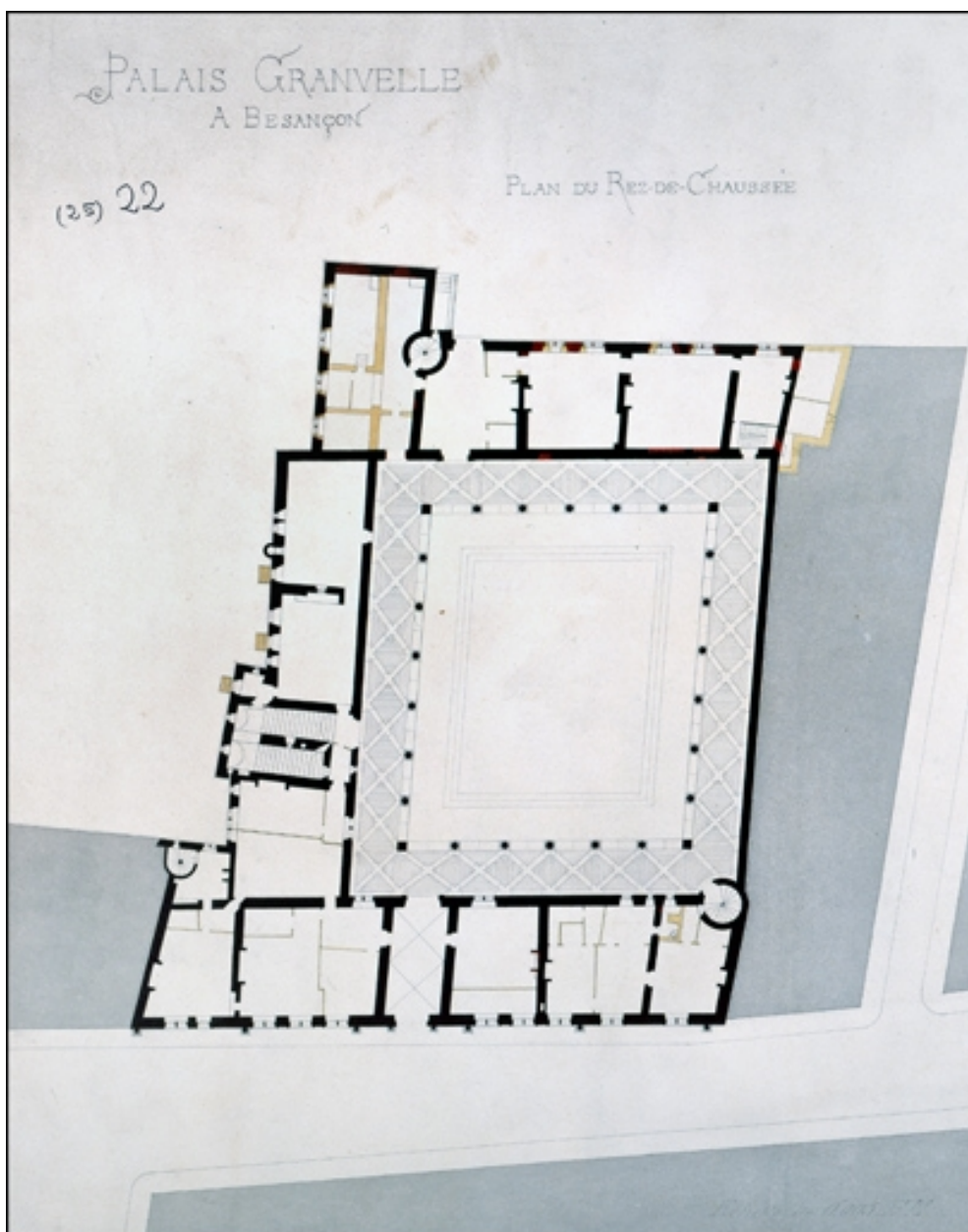
Plan du rez-de-chaussée. Dessin avec réhaut d'aquarelle, 1872.
