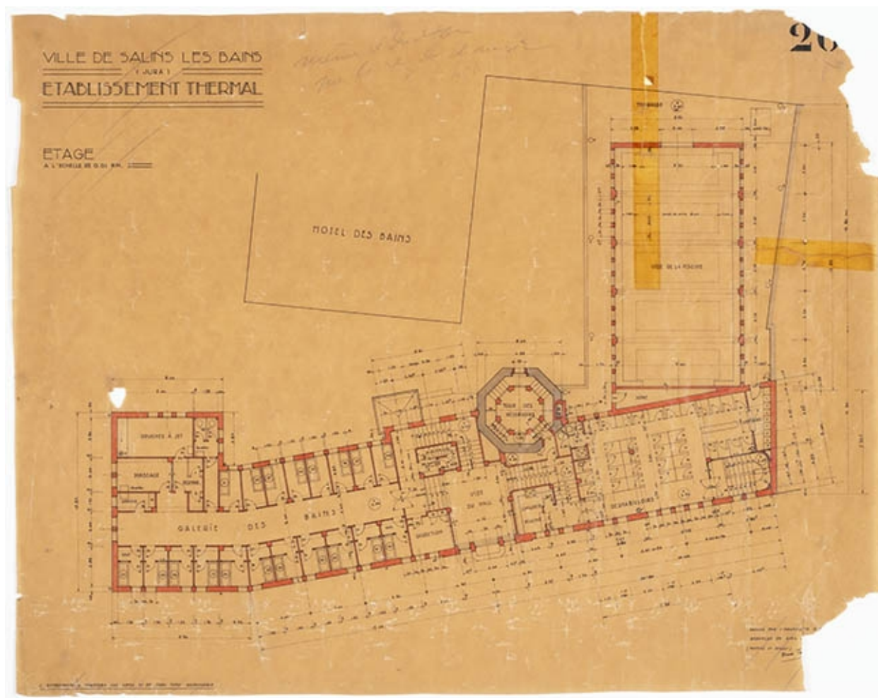
Projet de René Tournier (1934), plan du premier étage.
