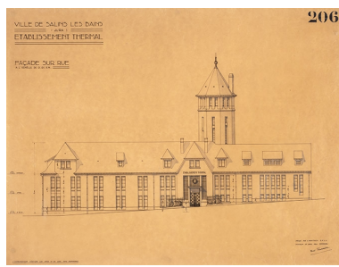
Projet de René Tournier (1934), façade sur la rue. Phot. Jérôme Mongreville, Autr. René Tournier IVR43_20213900156NUC4A
