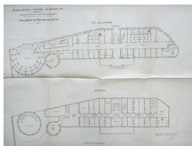
Plan du rez-de-chaussée et du premier étage (1917). Phot. Jérôme Mongreville, Autr. auteur inconnu IVR43_20223900086NUC4A
