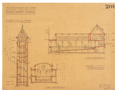
Projet de René Tournier (1934), coupes sur la piscine et la tour des réservoirs. Phot. Jérôme Mongreville, Autr. René Tournier IVR43_20213900159NUC4A
