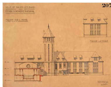
Projet de René Tournier (1934), façade sur la cour et coupe sur la piscine. Phot. Jérôme Mongreville, Autr. René Tournier IVR43_20213900157NUC4A
