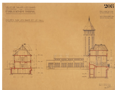
Projet de René Tournier (1934), façade sur la cour et coupe sur les bains. Phot. Jérôme Mongreville, Autr. René Tournier IVR43_20213900158NUC4A
