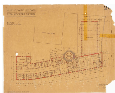
Projet de René Tournier (1934), plan du premier étage. Phot. Jérôme Mongreville, Autr. René Tournier IVR43_20213900153NUC4A
