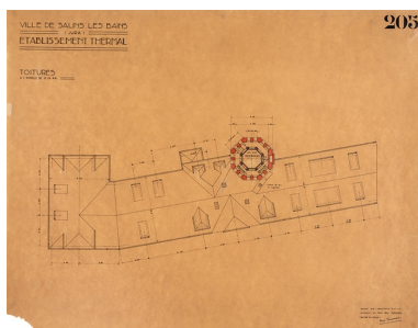
Projet de René Tournier (1934), plan des toitures. Phot. Jérôme Mongreville, Autr. René Tournier IVR43_20213900155NUC4A
