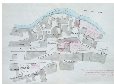
Plan-masse et de situation de l'établissement thermal (1883). Phot. Jérôme Mongreville, Autr. Claude Charles Chaffesey IVR43_20223900080NUC4A
