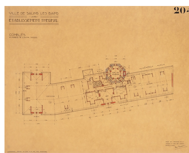
Projet de René Tournier (1934), plan des combles. Phot. Jérôme Mongreville, Autr. René Tournier IVR43_20213900154NUC4A
