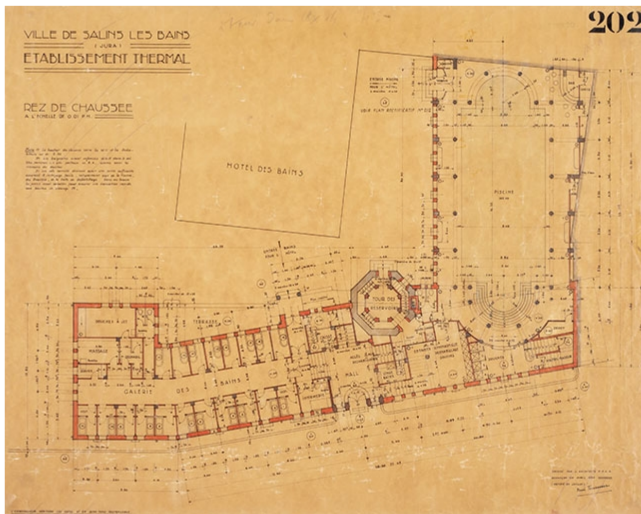
Projet de René Tournier (1934), plan du rez-de-chaussée.
