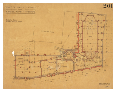
Projet de René Tournier (1934), plan du sous-sol. Phot. Jérôme Mongreville, Autr. René Tournier IVR43_20213900151NUC4A
