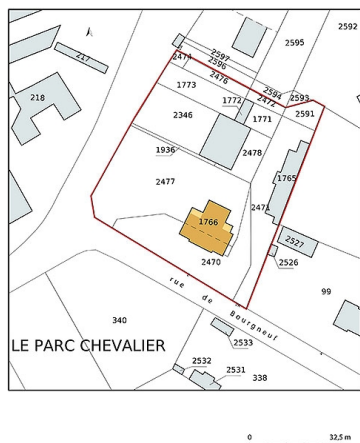
Plan-masse et de situation, extrait du plan cadastral (2021). Dess. Pierre-Marie Barbe-Richaud IVR26_20215800050NUDA
