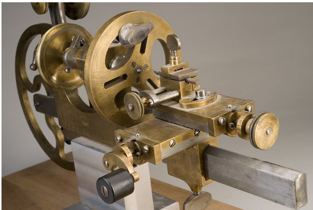
Chriot porte-outil et ensemble arbre-plateau (quill).
