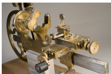
Chariot porte-outil et support de l'ensemble arbre-plateau (quill). Phot. Marc Loukachine IVR43_20122500081NUC4A
