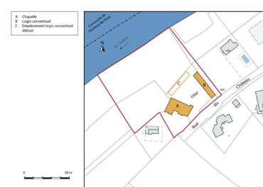
Plan masse de la chapelle et de l'ensemble conventuel Dess. Mathias Papigny IVR43_20167001415NUDA
