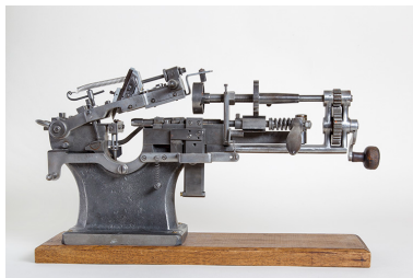
Vue de face. Phot. Jérôme Mongreville IVR43_20142500733NUC2A
