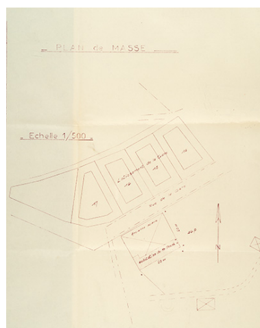
Monsieur Pronk Adrien à Damprichard – Doubs. Plan de masse, 26 juillet 1960. Phot. Jérôme Mongreville, Autr. Coopérative d'Etudes techniques rurales IVR43_20132500533NUC4A
