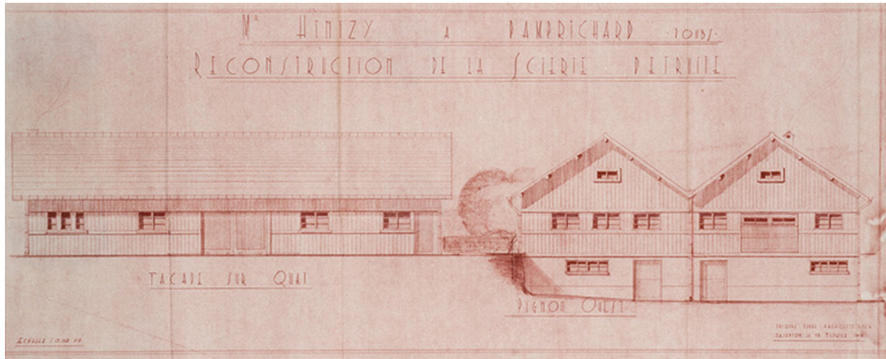
M Hintzi, sinistré à Damprichard – Doubs. Reconstruction de la scierie détruite. Façade sur quai [et] Pignon ouest, 18 février 1948.
