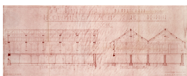
M Hintzy, sinistré à Damprichard – Doubs. Reconstruction de la scierie détruite. Coupes, 18 février 1948. Phot. Jérôme Mongreville, Autr. Jacques Duval IVR43_20132500542NUC4A
