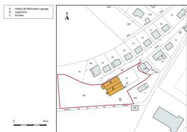
Plan-masse et de situation. Extrait du plan cadastral, 2012, section AB. Dess. Mathias Papigny IVR43_20142501514NUDA
