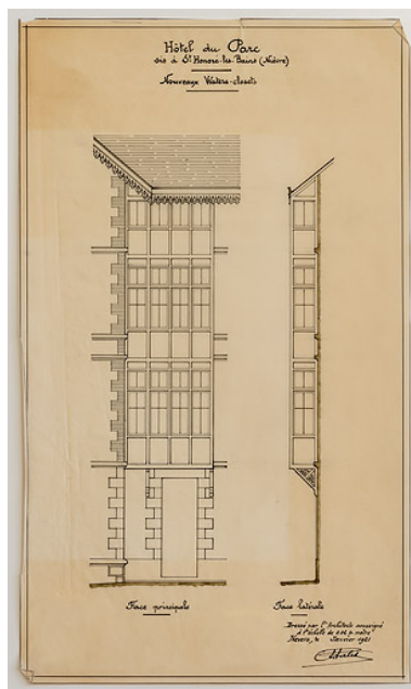
Oriel en surplomb de la façade côté pour les water-closet (1921), élévations. Repro. Pierre-Marie Barbe-Richaud, Autr. Auguste Palet IVR26_20205800120NUC4A
