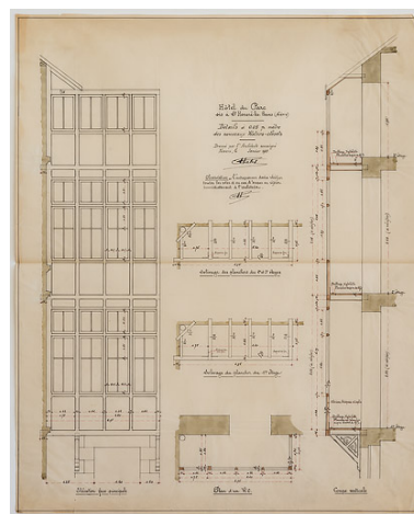
Oriel en surplomb de la façade côté pour les water-closet (1921), plan, élévation et coupe. Repro. Pierre-Marie Barbe-Richaud, Autr. Auguste Palet IVR26_20205800125NUC2A
