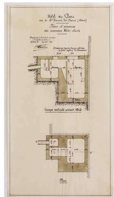
Fosse d'aisances, plan et coupe. Repro. Pierre-Marie Barbe-Richaud, Autr. Auguste Palet IVR26_20205800126NUC2A
