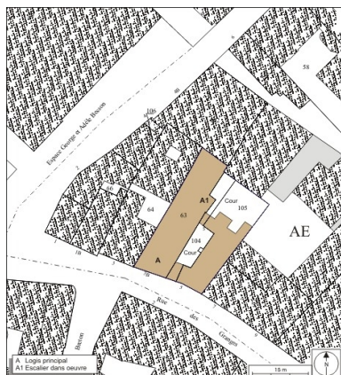
Plan masse et de situation. Extrait du plan cadastral, 1974, section AE Dess. André Céréza IVR43_20102500067NUDA
