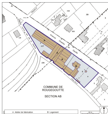
Plan-masse et de situation. Montage d'extraits de plan cadastral, Giromagny, 1984, section AI, 1:1000 et Rougegoutte, 1983, section AH, 1:1000. Dess. André Céréza IVR43_20039000051NUDA
