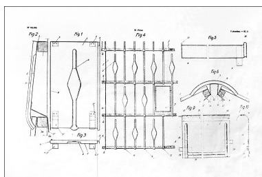
[Tuiles standard, faîtière et de rive], 1946. IVR43_20093900001NUC2A
