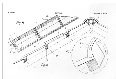
[Tuiles faîtière et de rive, et exemple d'assemblage sur toiture], 1946. IVR43_20093900002NUC2A
