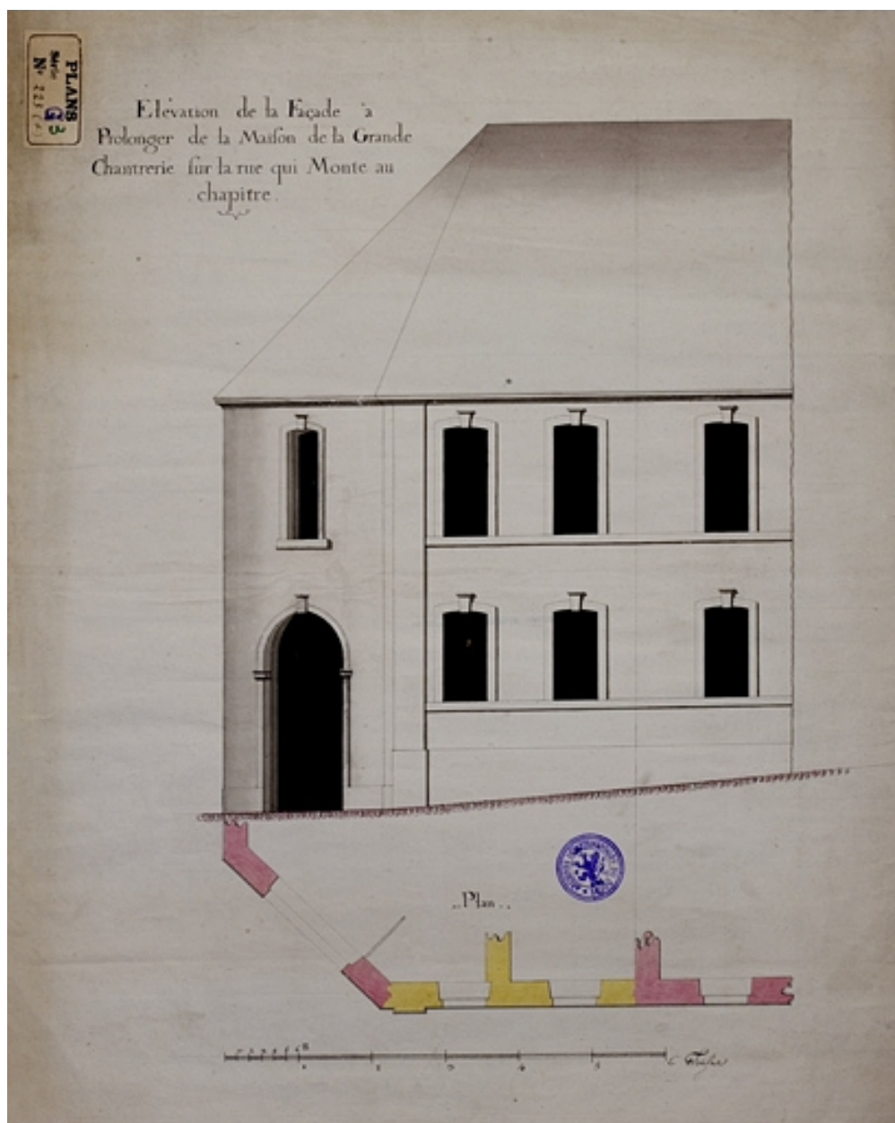
Elévation de la façade à prolonger de la maison de la Grande Chantrerie sur la rue qui monte au Chapitre. Dessin à la plume et aquarelle, 1783.
