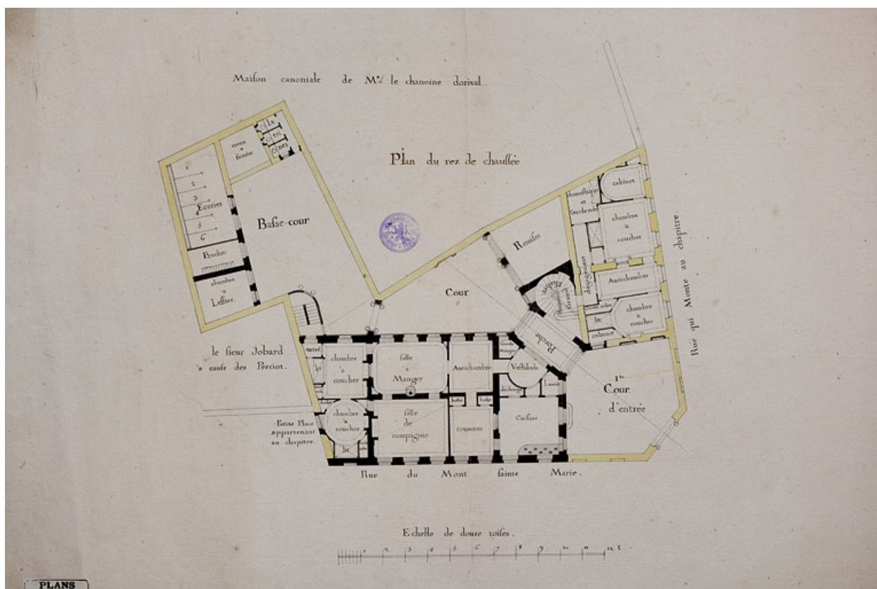
Plan du rez-de-chaussée : nouvelle distribution. Dessin à la plume et aquarelle, 1783.
