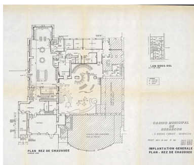
État des lieux, plan du rez-de-chaussée (1993).
