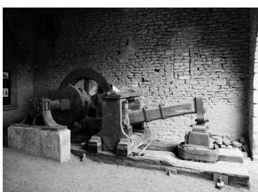
Forge d'affinerie, halle d'entrée, martinet de platinerie. Phot. Jean-Luc Duthu IVR26_19932100912V
