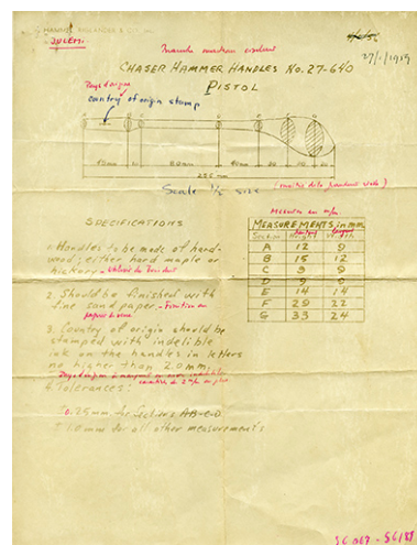
Dessin technique d'un manche de marteau de ciseleur envoyé par la société Hammel, Riglander & Co, 27 janvier 1959. Phot. Sonia Dourlot IVR43_20172500742NUC4A
