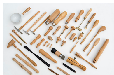
Exemples de manches fabriqués par Félix et Gabriel Coulot. Phot. Sonia Dourlot IVR43_20172500738NUC4A
