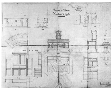
Ameublement de l'église : plan des stalles du chœur, bancs de
