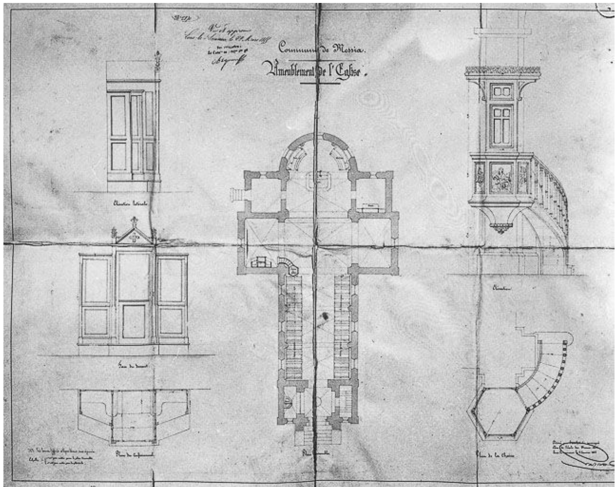
Ameublement de l'église : plan de la chaire et du confessionnal, 1855.
