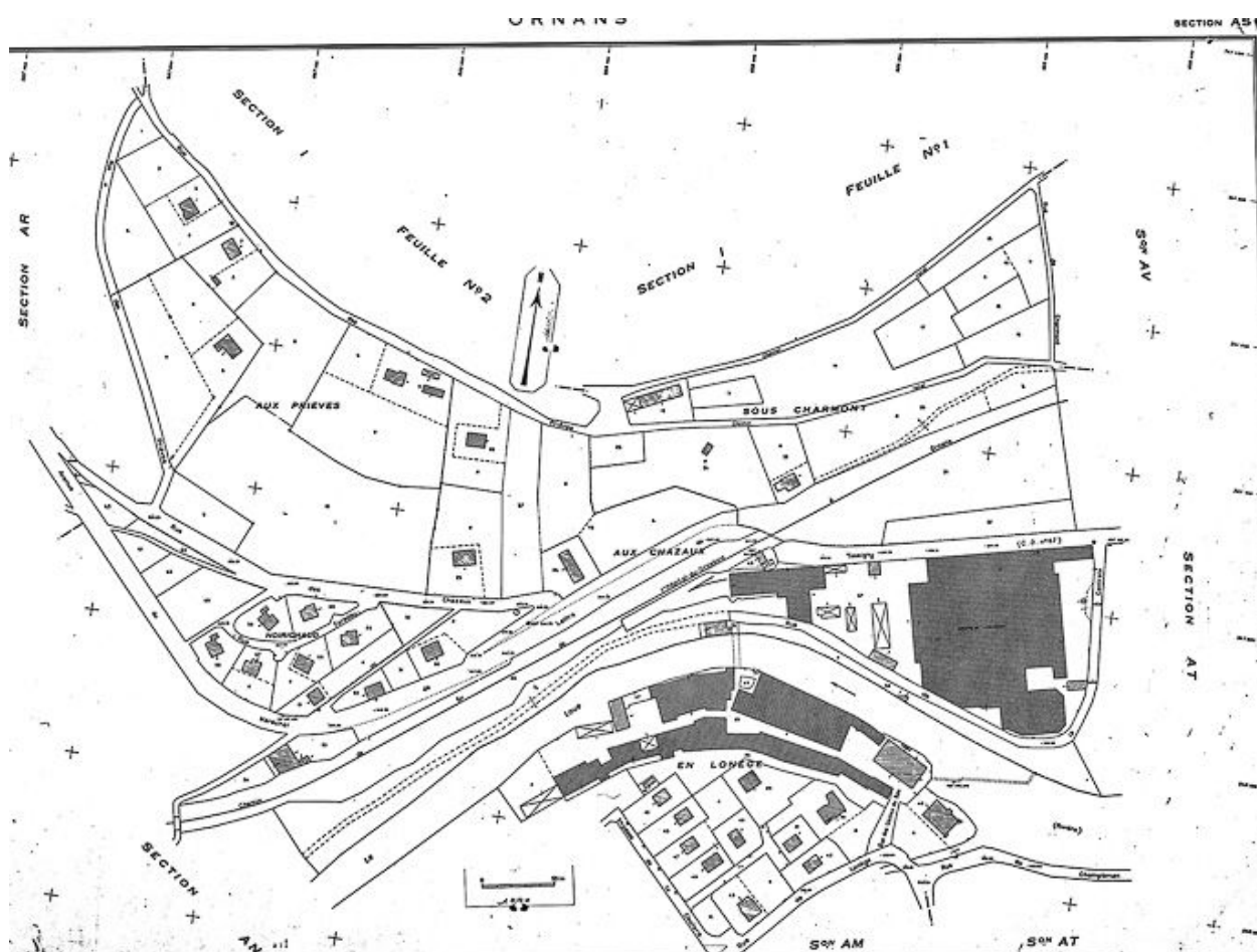
Plan cadastral, 1975, section AS, échelle 1 : 500.
