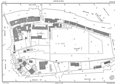
Plan cadastral, 1975, section AD, échelle 1 : 500.
