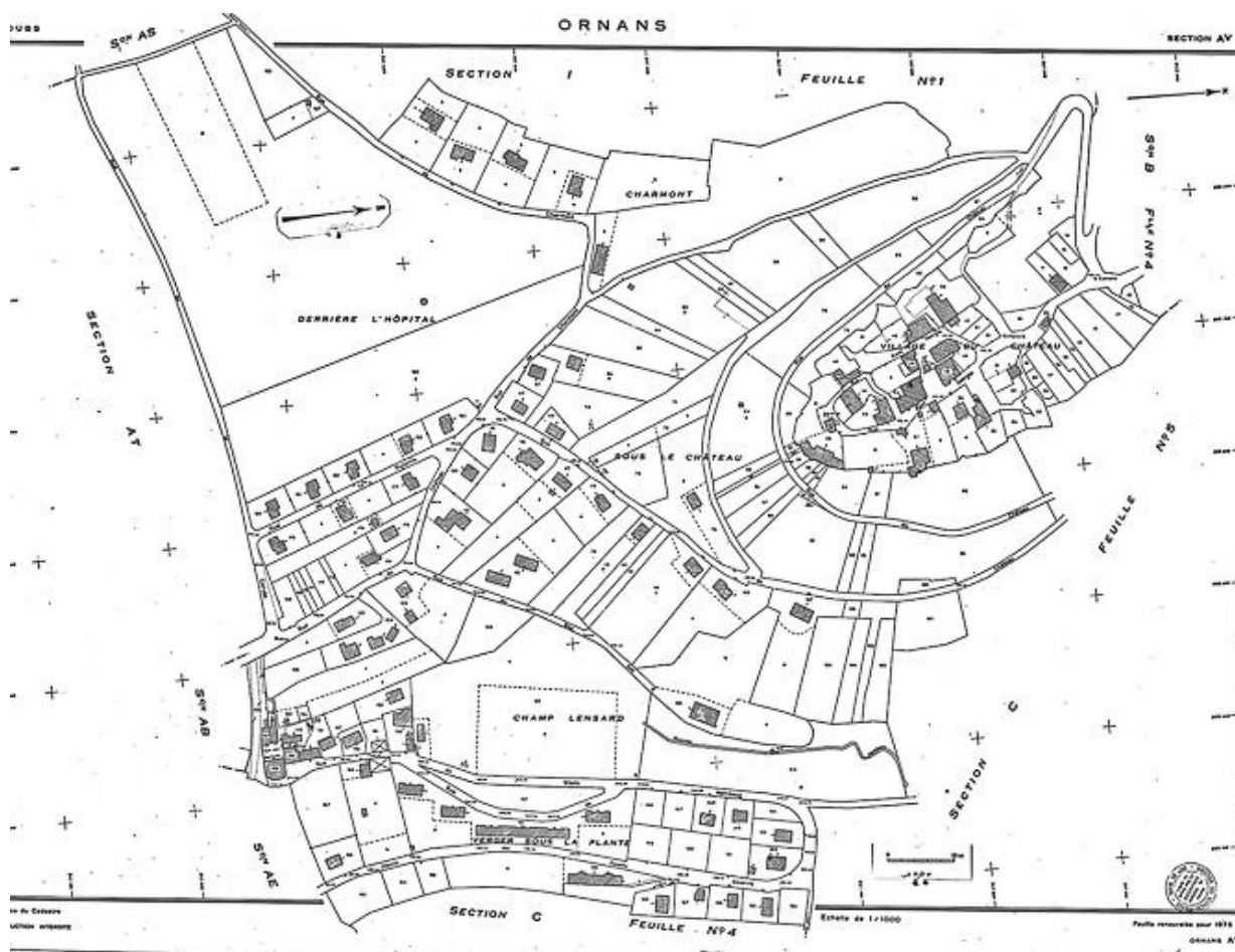
Plan cadastral, 1975, section AV, échelle 1 : 1000.
