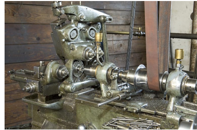
Tour à décolleter Petermann (M). Détail du système d'entraînement de la poupée mobile. Phot. Jérôme Mongreville IVR43_20082500031NUC2A
