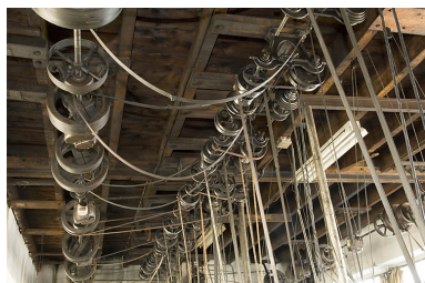
Poulies et courroies en cuir du système de transmission. Phot. Jérôme Mongreville IVR43_20082500026NUC2A
