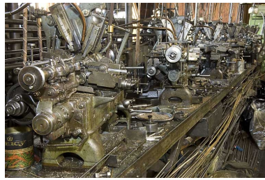
Alignement des tours à décolleter Petermann (M). Phot. Jérôme Mongreville IVR43_20082500030NUC2A
