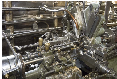
Détail des outils de coupe d'un tour à décolleter Petermann (M). Phot. Jérôme Mongreville IVR43_20082500035NUC2A
