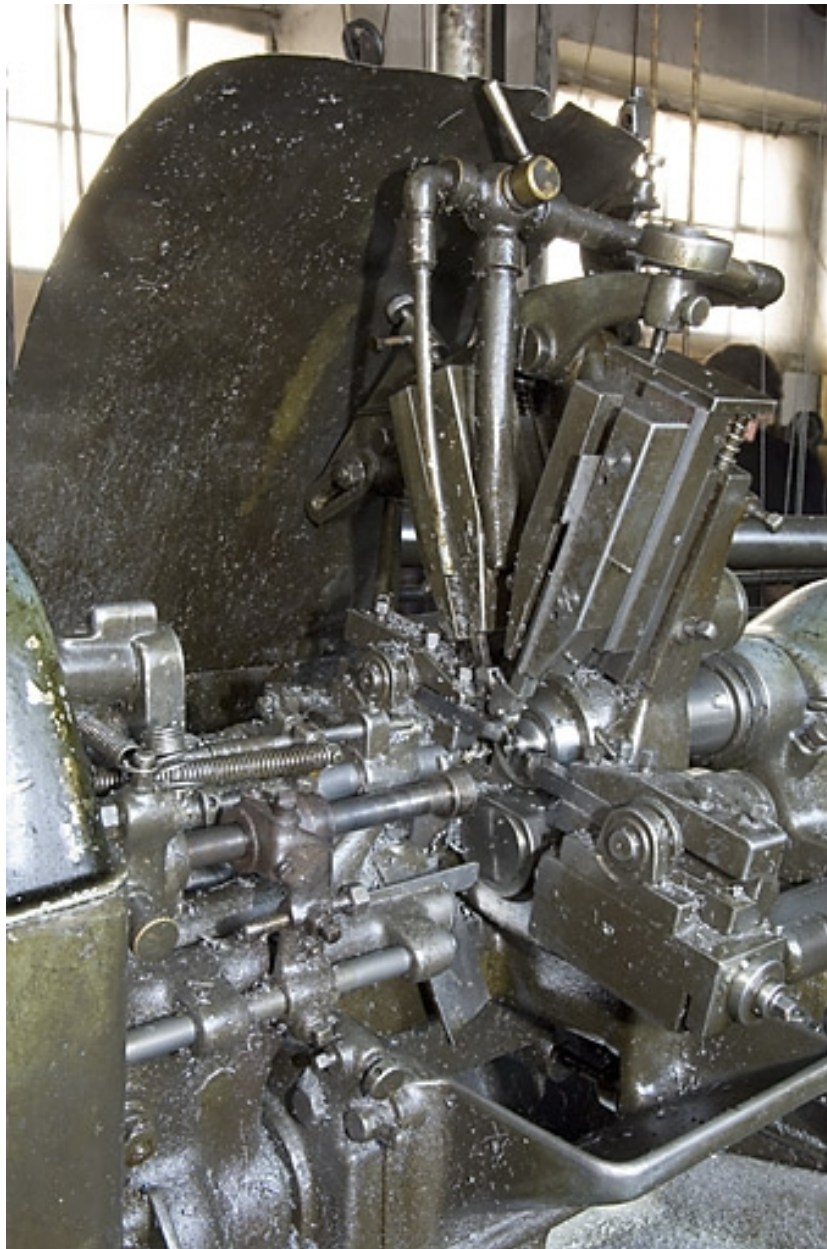
Tour à décolleter 2 A Jos. Petermann (J). Détail.
