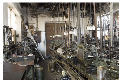
Atelier de fabrication : machines- outils et éléments de transmission. Phot. Jérôme Mongreville IVR43_20082500023NUC2A
