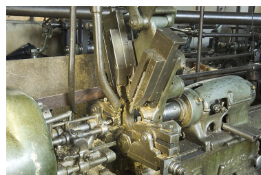
Tour à décolleter 10 HS Jos. Petermann (K). Détail. Phot. Jérôme Mongreville IVR43_20082500021NUC2A
