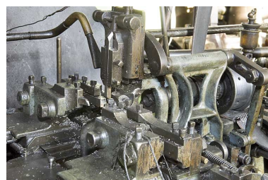
Tour à décolleter Beldi (L). Détail. Phot. Jérôme Mongreville IVR43_20082500056NUC2A
