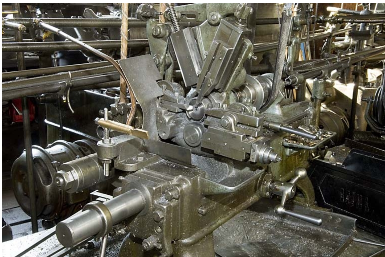
Tour à décolleter Petermann (M). Détail des outils de coupe (au centre).
