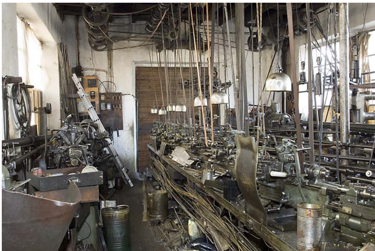
Atelier de fabrication : machines-outils et éléments de transmission.
