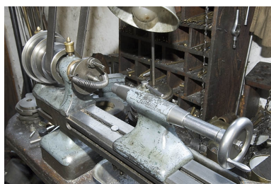
Tour horizontal Waltham (B). Détail de la poulée fixe et de la poulée mobile. Phot. Jérôme Mongreville IVR43_20082500042NUC2A
