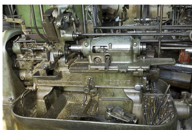
Tour à décolleter 10 HS Jos. Petermann (K). Phot. Jérôme Mongreville IVR43_20082500022NUC2A
