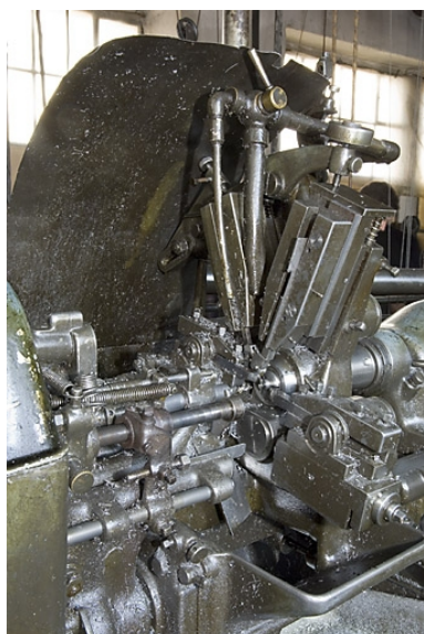
Tour à décolleter 2 A Jos. Petermann (J). Détail. Phot. Jérôme Mongreville IVR43_20082500020NUC2A
