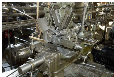
Tour à décolleter Petermann (M). Détail des outils de coupe (au centre). Phot. Jérôme Mongreville IVR43_20082500032NUC2A
