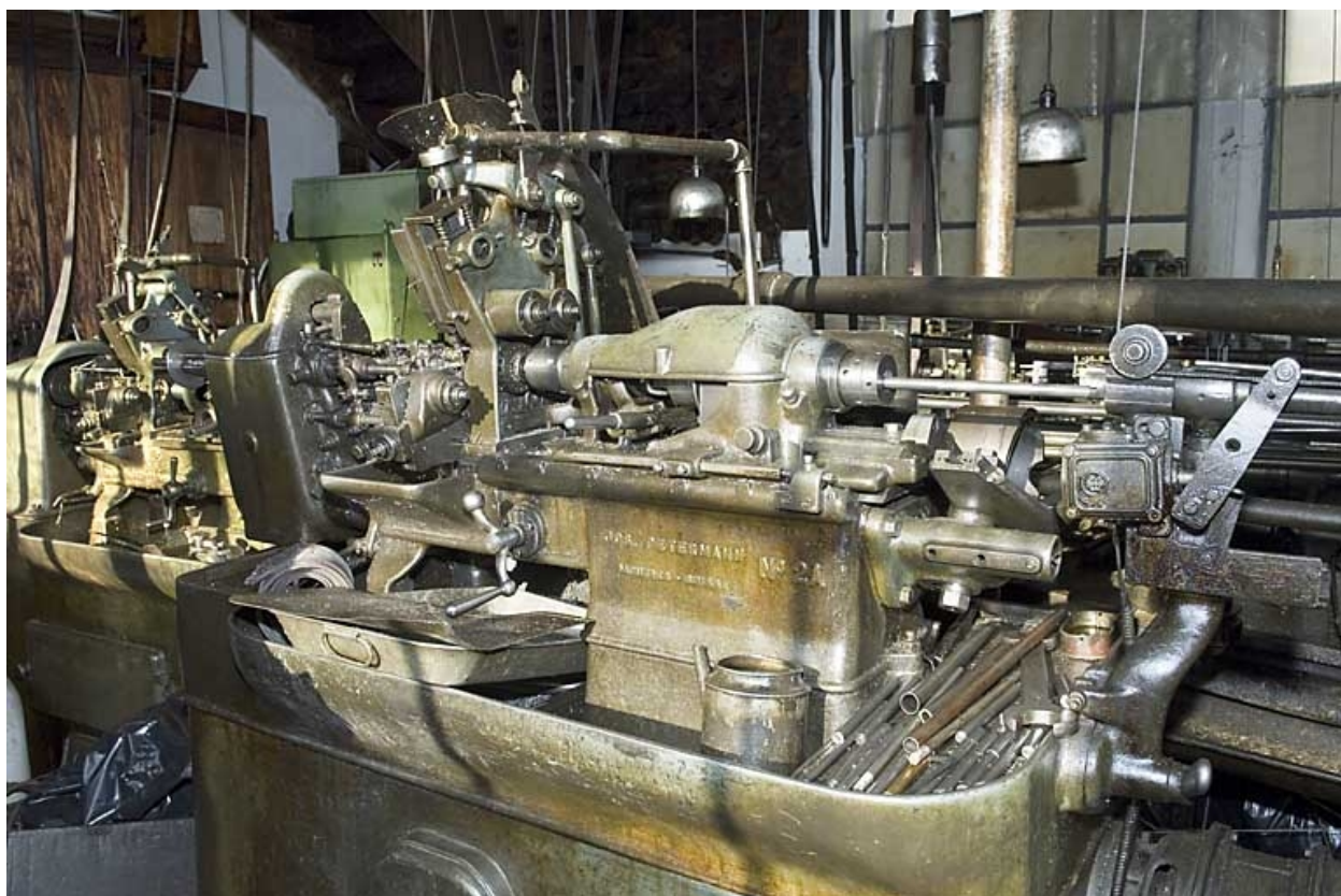
Tour à décolleter 2 A Jos. Petermann (J).
