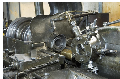
Tour à décolleter Loewe & Co (N). Détail du barillet porte-outils. Phot. Jérôme Mongreville IVR43_20082500037NUC2A
