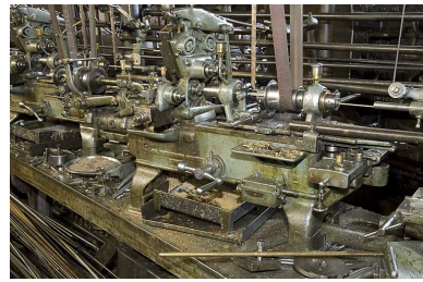
Tour à décolleter Petermann (M). Phot. Jérôme Mongreville IVR43_20082500033NUC2A
