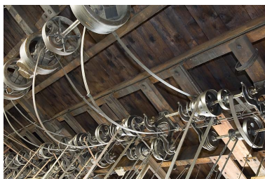
Les arbres de transmission équipés des poulies et des courroies. Phot. Jérôme Mongreville IVR43_20082500027NUC2A
