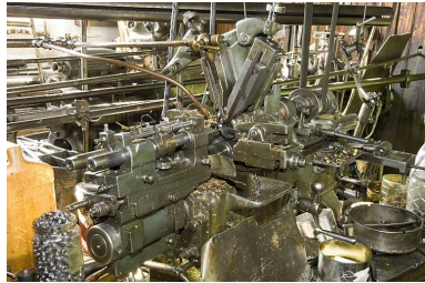
Détail d'un tour à décolleter Petermann (M). Phot. Jérôme Mongreville IVR43_20082500034NUC2A
