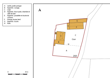
Plan-masse et de situation. Extrait du plan cadastral, 2018, section B, 1/1000. Dess. Bertrand Turina IVR26_20207100168NUDA
