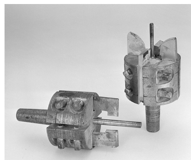
Détail de deux outils de coupe. Phot. Jérôme Mongreville IVR43_20022500951X
