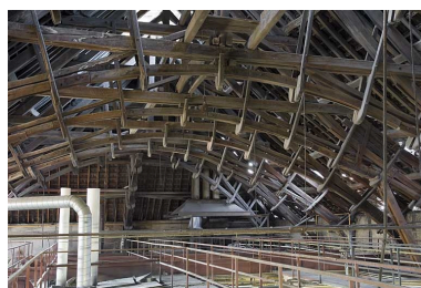
Charpente de l'atelier des fours. Détail des fermes. Phot. Jérôme Mongreville IVR43_20077000931NUCA
