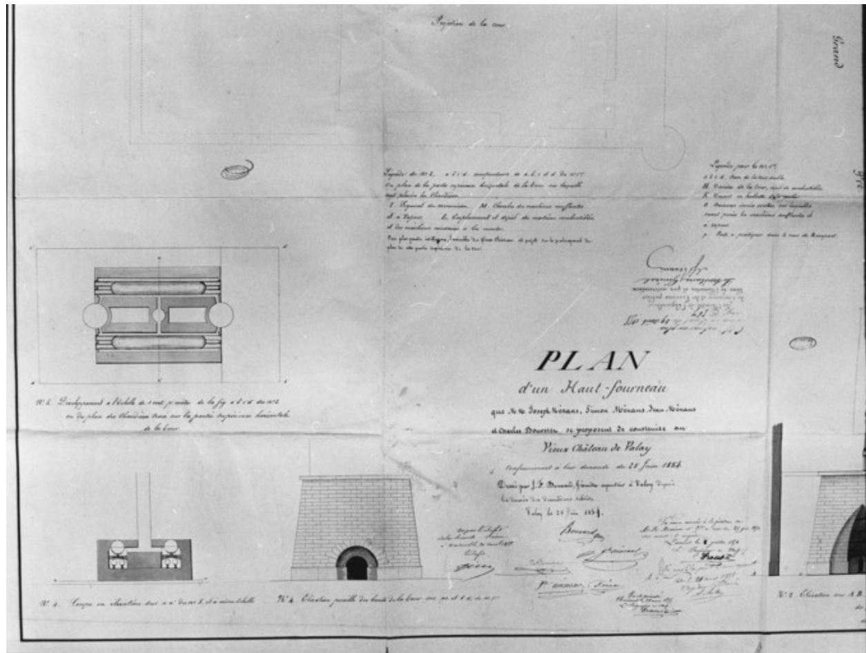
Plan d'un haut-fourneau que MM. [...] se proposent de construire au Vieux Château de Valay [détail de la partie gauche : plan, coupe et élévation].
