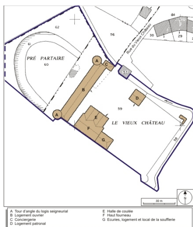
Plan-masse et de situation. Extrait du plan cadastral numérisé, 2008, section AC, 1:1000. Source : Direction générale des Finances Publiques - Cadastre ; mise à jour : 2008. Dess. André Céréza IVR43_20087000496NUDA
