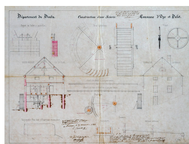
Moulin et scierie communale, Oye-et-Pallet : construction d'une scierie [Elévation, coupe et détails], 1848. Phot. Jérôme Mongreville IVR43_20182500118NUC4A
