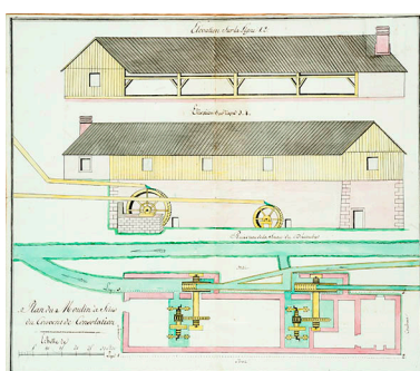
Scierie, Consolation-Maisonnettes (Val de Consolation) : plan du moulin à scies du couvent de Consolation, s.d. [vers 1820]. Phot. Jérôme Mongreville IVR43_20152500577NUC4A
