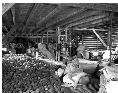
Usine de tabletterie (usine de pipes) Chapuis-Comoy, Saint-Claude (2-4 rue des Etapes) : intérieur du séchoir à ébauchons (rue des Petites Etapes). Phot. Jérôme Mongreville IVR43_19923900489X
