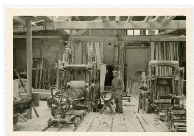
Scierie Gaiffe, Montlebon (Cornabey) : [les châssis de scie multilames], années 1950-1960. Autr. auteur inconnu
