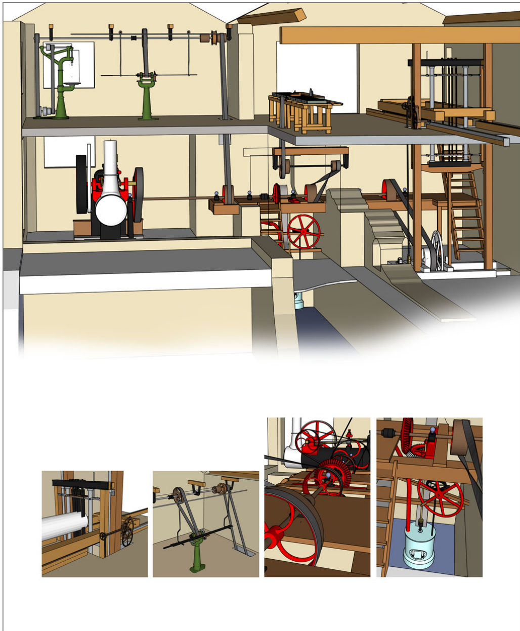
Moulin et scierie Donzé puis Lescot, Rémondans-Vaivre : schéma de distribution de la force motrice.
