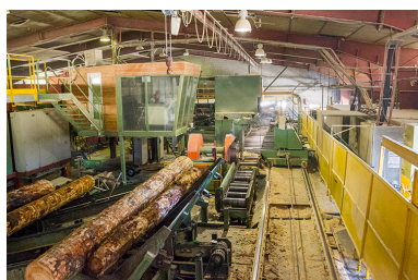
Scierie Thidric puis Gaume ou Grande Scierie mécanique de Maîche, Maîche : ligne ruban, pour les commandes diversifiées. Phot. Yves Sancey IVR43_20132501732NUC2A
