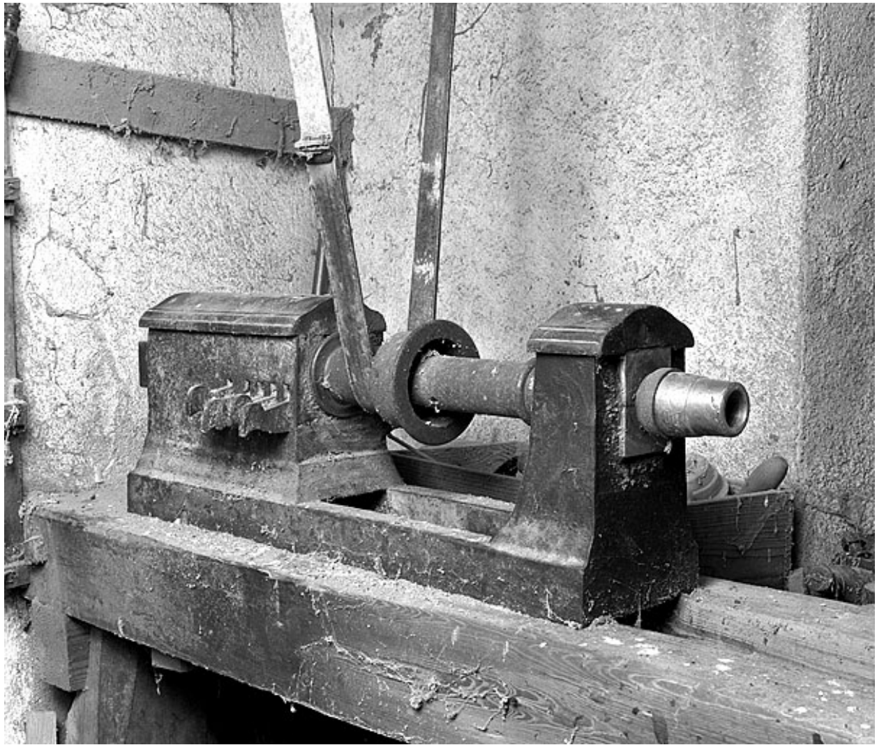
Usine de tabletterie (tournerie) Vuillermoz, Vulvoz (au Moulin) : tour à bois Lartaux (Saint-Claude).
