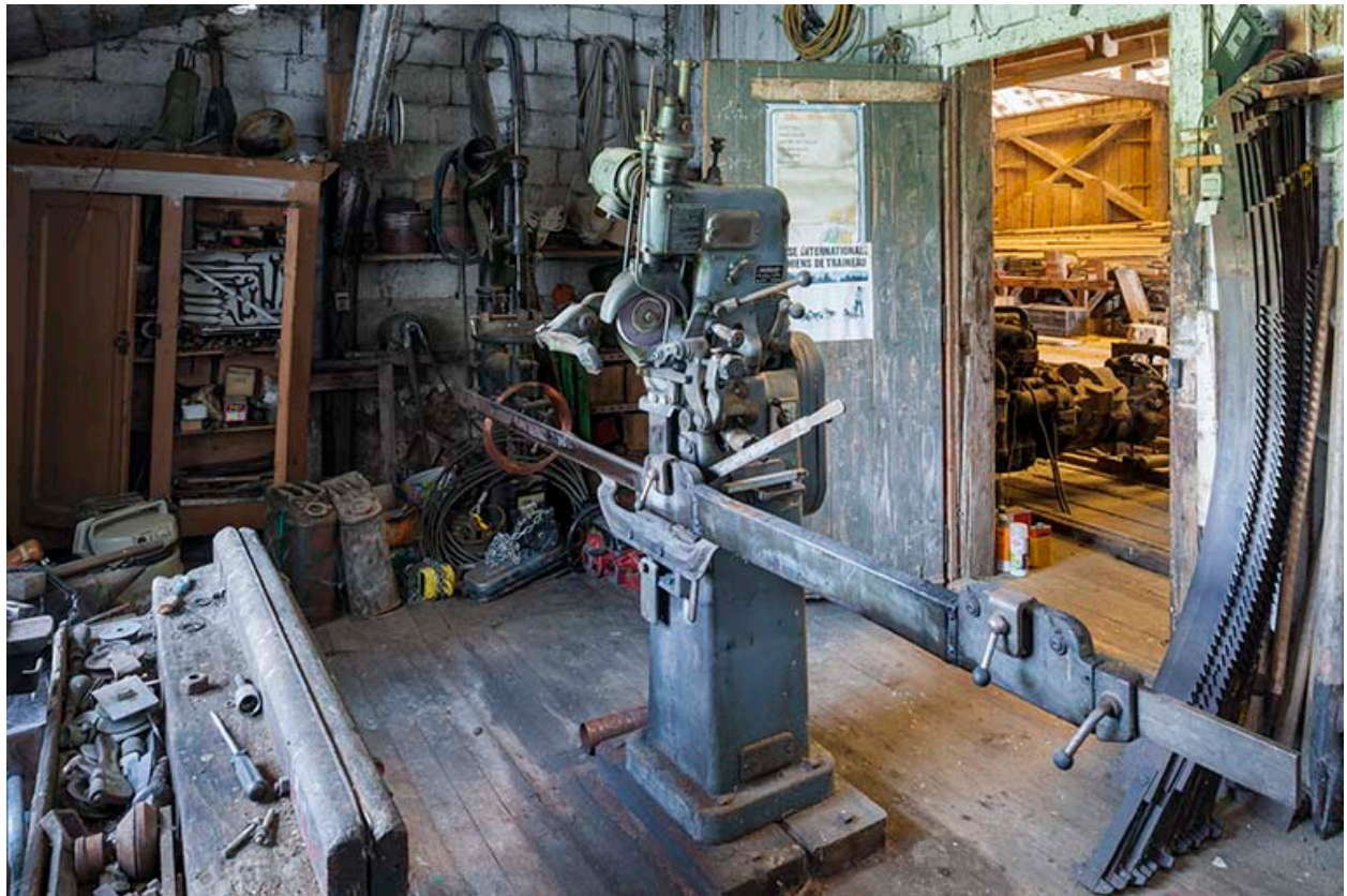
Scierie Thiébaud, Labergement-Sainte-Marie : atelier d'affûtage.
