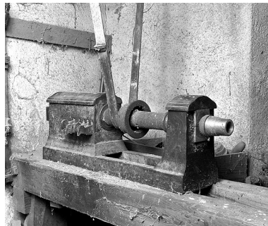
Usine de tabletterie (tournerie) Vuillermoz, Vulvoz (au Moulin) : tour à bois Lartaux (Saint-Claude). Phot. Jérôme Mongreville IVR43_19943901196X
