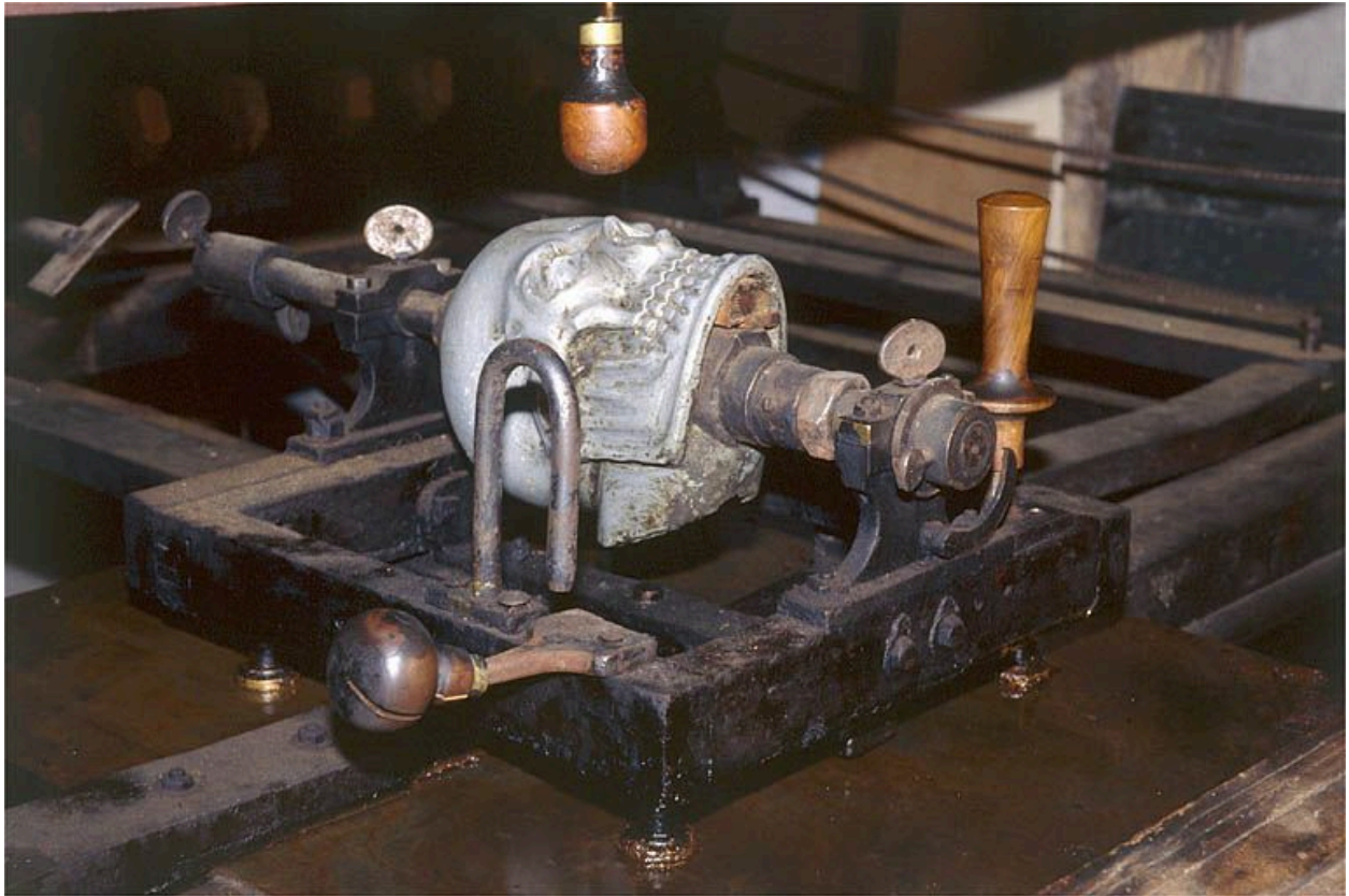
Machine à sculpter les têtes de pipes de l'atelier d'Olivier Racine, Saint-Claude (Etables) : modèle et son support.
