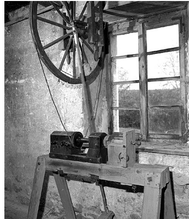
Tour à bois (tour à marchepied). Phot. Jérôme Mongreville IVR43_19943901208X
