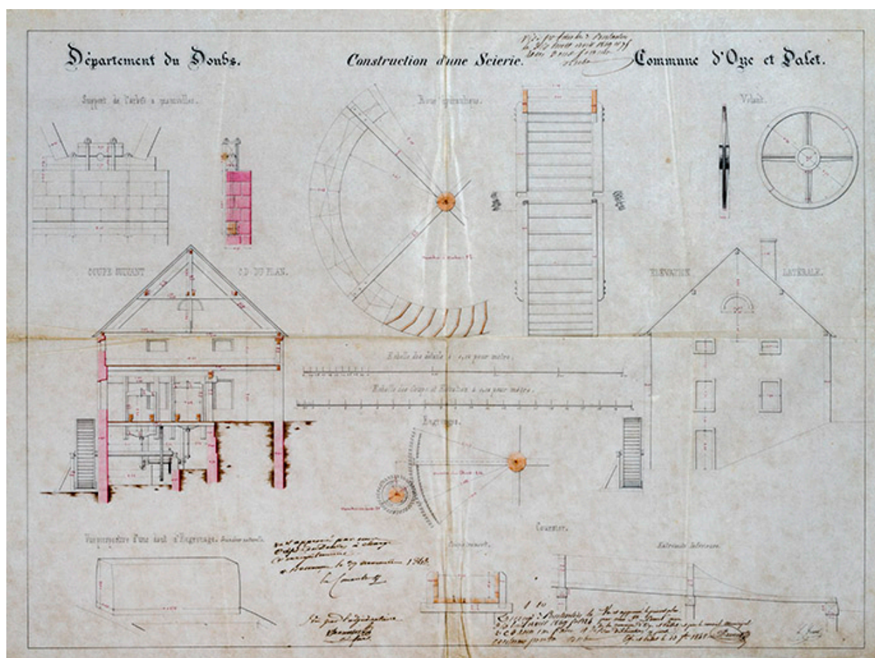
Moulin et scierie communale, Oye-et-Pallet : construction d'une scierie [Elévation, coupe et détails], 1848.
