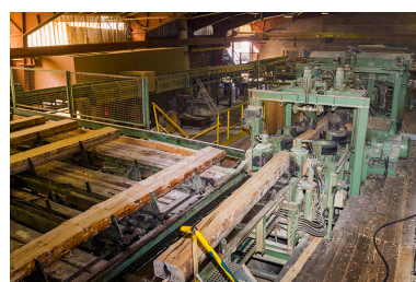
Scierie Thidric puis Gaume ou Grande Scierie mécanique de Maîche, Maîche : ligne "canter", pour les commandes destinées à la grande distribution. Phot. Yves Sancey IVR43_20132501730NUC2A
