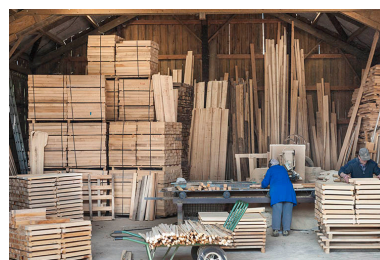
Moulin des Calots, actuellement scierie Stofleth, Sancey-le- Long : mise sur palettes des palettes des pièces découpées. Phot. Jérôme Mongreville IVR43_20152500426NUC4A
