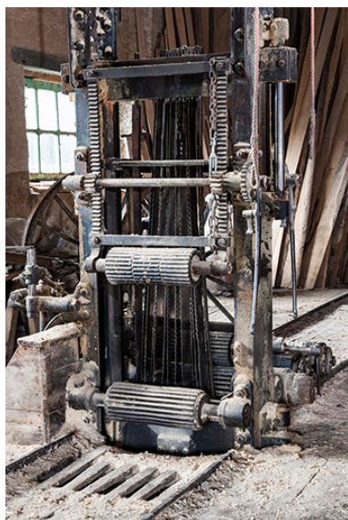
Scierie des Mortes, Chapelle-des-Bois (les Mortes) : châssis de scie multilame Benier-Rollet. Phot. Jérôme Mongreville IVR43_20152501802NUC4A
