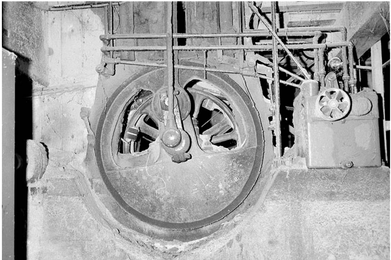
Usine de tournerie et scierie Janier-Vuillermoz, Lavans-lès-Saint-Claude (2-4 rue du Caton) : système d'entrainement du châssis de scie multilame Socolest.
