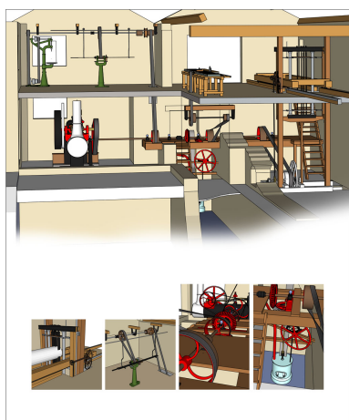
Moulin et scierie Donzé puis Lescot, Rémondans-Vaivre : schéma de distribution de la force motrice. Dess. Mathias Papigny IVR43_20142500590NUDA
