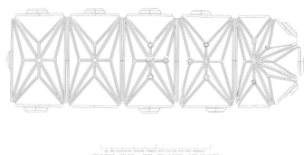
Plan du couvrement. IVR26_20122100826A2YY
