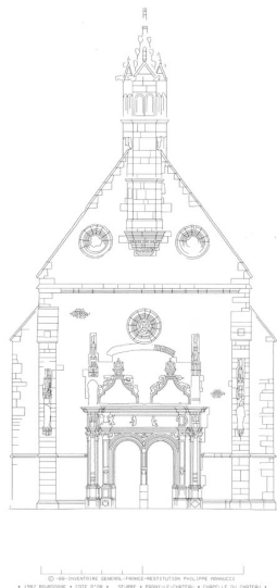
Façade principale. Dess. Alain Morelière, Dess. Philippe Manucci, Dess. A.P.A.I.G (Atelier de photogrammétrie architecturale de l'Inventaire général) IVR26_20122100828A2YY
