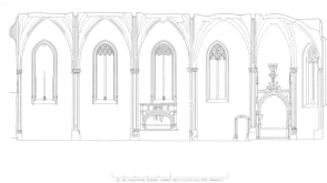
Coupe longitudinale. Dess. Alain Morelière, Dess. Philippe Manucci, Dess. A.P.A.I.G (Atelier de photogrammétrie architecturale de l'Inventaire général) IVR26_20122100825A2YY
