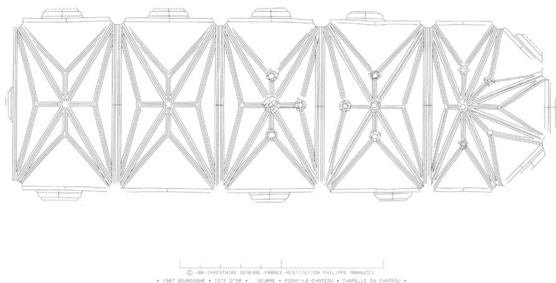
Plan du couvrement.
