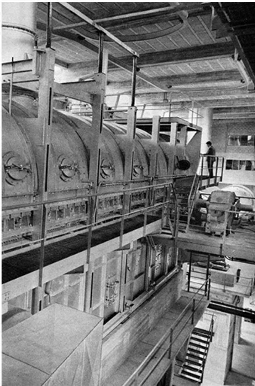
Four rotatif : zone de décarbonatation.
