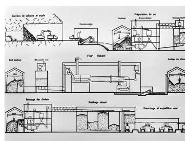
Chaîne de fabrication avec four rotatif. Phot. Jérôme Mongreville IVR43_19973900937X
