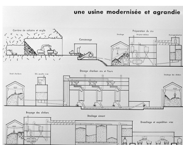
Chaîne de fabrication avec fours verticaux. Phot. Jérôme Mongreville IVR43_19973900936X
