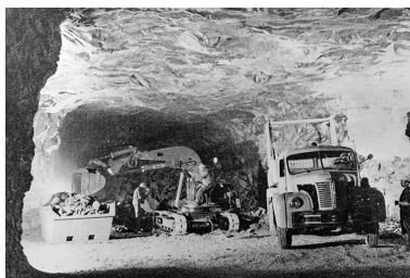
Chargement et évacuation du calcaire. Phot. Jérôme Mongreville IVR43_19973900951X
