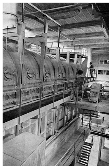
Four rotatif : zone de décarbonation. Phot. Jérôme Mongreville IVR43_19973900960X
