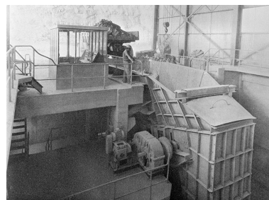
Poste de concassage en carrière avec évacuation sur l'usine par bande transporteuse. Phot. Jérôme Mongreville IVR43_19973900944X
