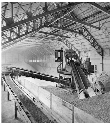
Hall de stockage et de manutention. Phot. Jérôme Mongreville IVR43_19973900935X
