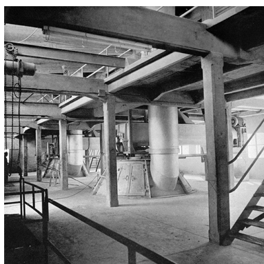
Etage supérieur des fours. Phot. Jérôme Mongreville IVR43_19973900965X
