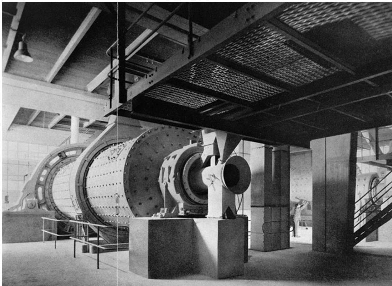
Atelier des broyeurs.
