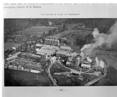
Vue aérienne de l'usine de Champagnole. Phot. Jérôme Mongreville IVR43_19963900403X
