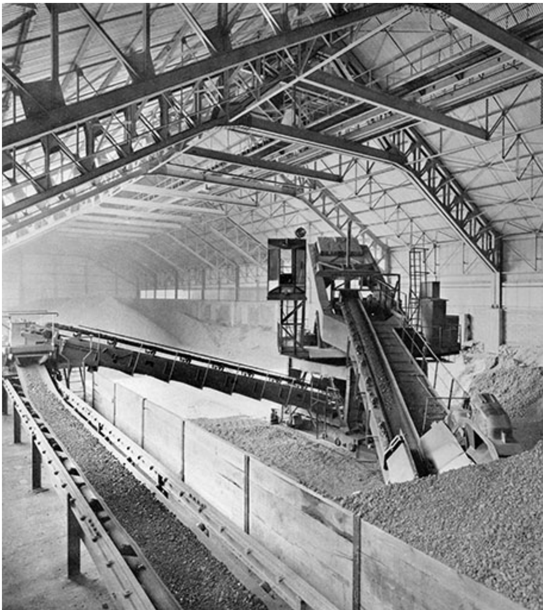
Hall de préhomogénéisation.
