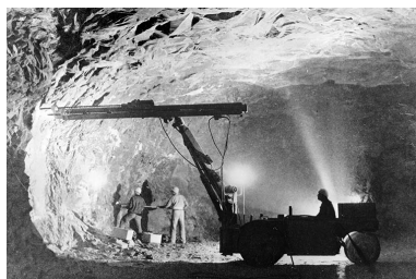
Carrière - Minage avec perforatrice sur jumbo. Phot. Jérôme Mongreville IVR43_19973900950X
