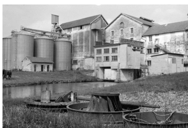
Bâtiment d'eau (J), ateliers de fabrication (L, M) et silos (C, D) vus du sud-ouest.Éléments d'une turbine Singrun au premier plan.
