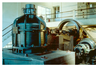
Bâtiment d'eau : réducteur Messian et dynamo de la Cie Générale Electricque.
