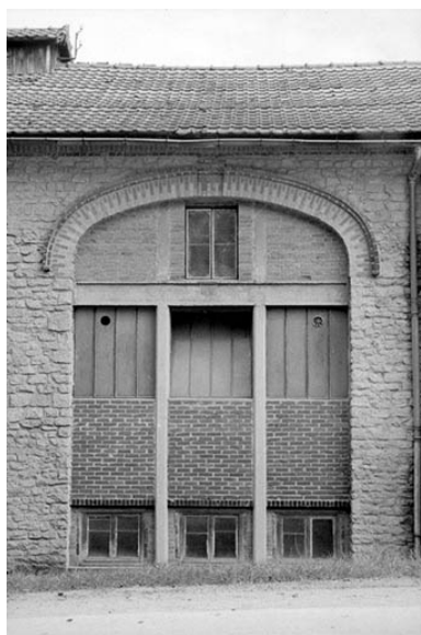
Atelier (A) : détail d'une travée large. Phot. Laurent Poupard IVR43_19893900047Z
