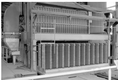
Atelier (M) : four à bassin en cours de chargement. Phot. Laurent Poupard IVR43_19893900058Z
