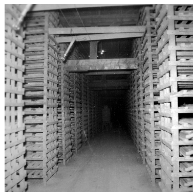
Le séchoir et ses "perchets". Phot. Jérôme Mongreville IVR43_19893900064X
