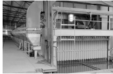
Atelier (M) : four à bassin. Phot. Laurent Poupard IVR43_19893900057Z
