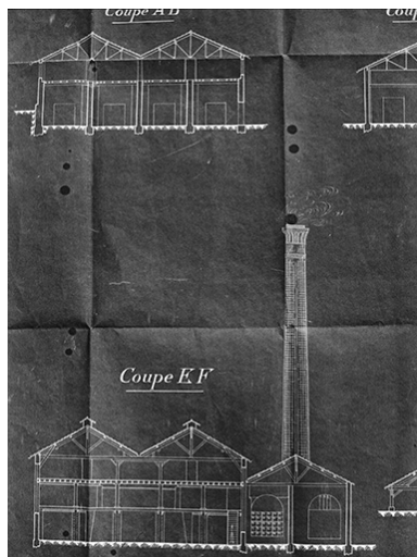
Coupe transversale de l'atelier de fabrication (A). Phot. Jack Dumont IVR43_19793900404Z
