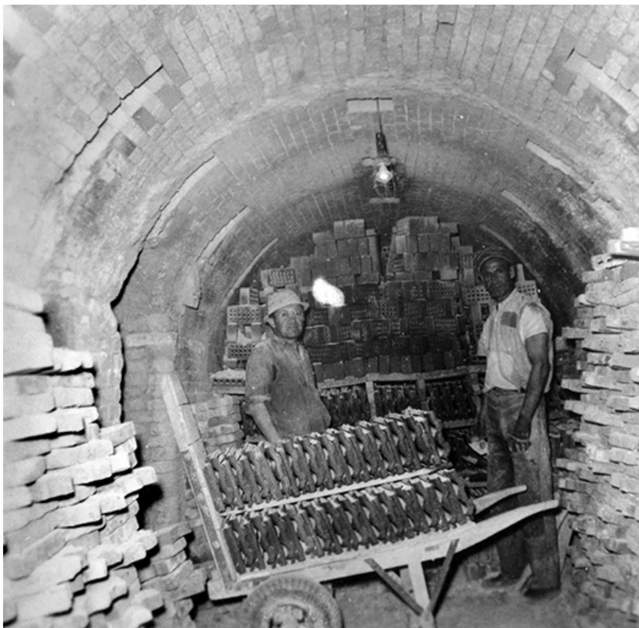
Déchargement du four Hoffmann.
