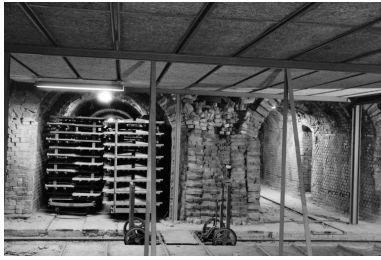
Atelier (A) : ancien four Hoffmann (dû à la société Simon). Phot. Laurent Poupard IVR43_19893900052Z
